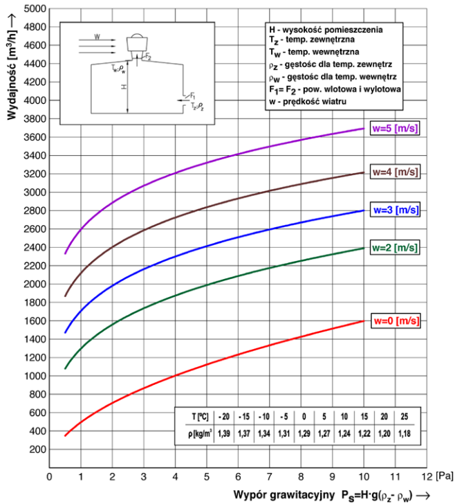
Charakterystyka przepływowa wywiewtrzaka zespolonego W-z 630/WDc/s-31,5 i W-z 630/WDc/sw-31,5 w zależności od wyporu grawitacyjnego i prędkości wiatru
