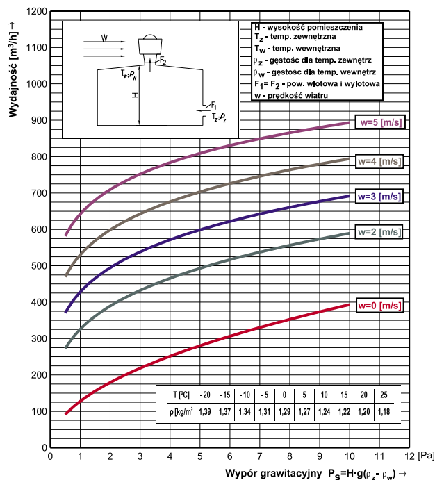
Charakterystyka przepływowa wywiewtrzaaka zespolonego W-z 315/WDc/s-16 i W-z 315/WDc/sw-16 w zależności od wyporu grawitacyjnego i prędkości wiatru.
