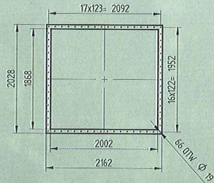
WYLOT OBUDOWA/KOMPENSATOR
