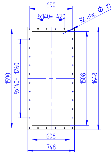
WLOT WLOT KOLANOWY
