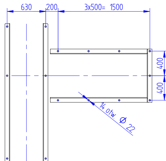
ROZMIESZCZENIE OTWORÓW POD ŚRUBY FUNDAMENTOWE
