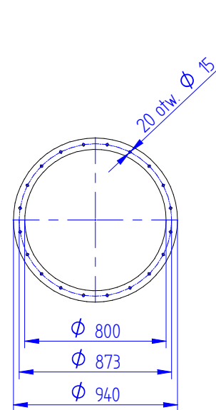
WLOT KROCIĆ WLOTOWY
