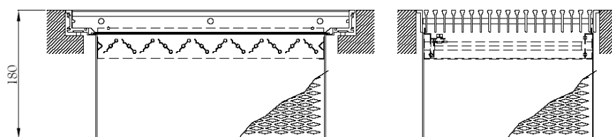
Kratka UP0-AT z ramką montażową i regulacją wysokości oraz przepustnicą SCUP i skrzynką rozprężną
