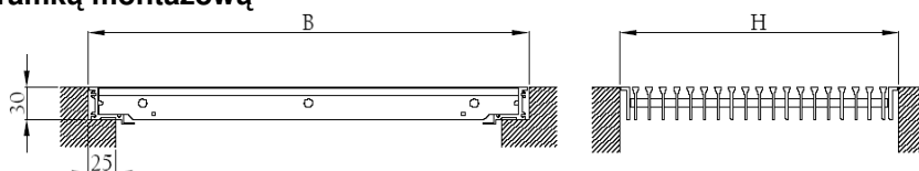
Kratka UP0-AC z ramką montażową
