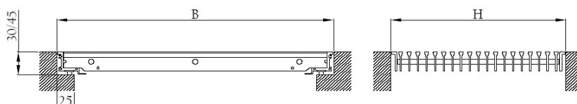
Kratka UP0-AT z ramką montażową i regulacją wysokości
