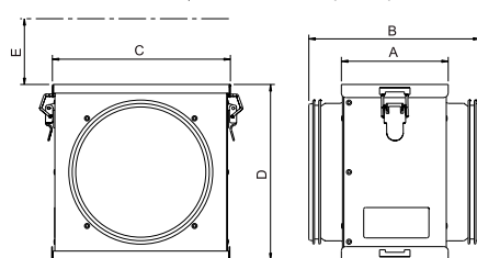
Minimalna wolna przestrzeń do wymiany filtra
