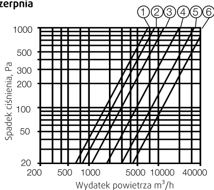
LGH – Czerpnia
