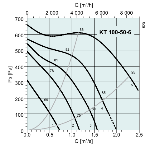
Min. przeciwnieśnienie stat.: 250 Pa
