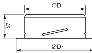
Rysunek 3. Kotnierz montażowy.
