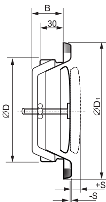
Rysunek 2. Zawór wywiewny KK.
