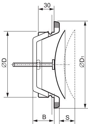
Rysunek 1. Zawór nawiewny KE.
