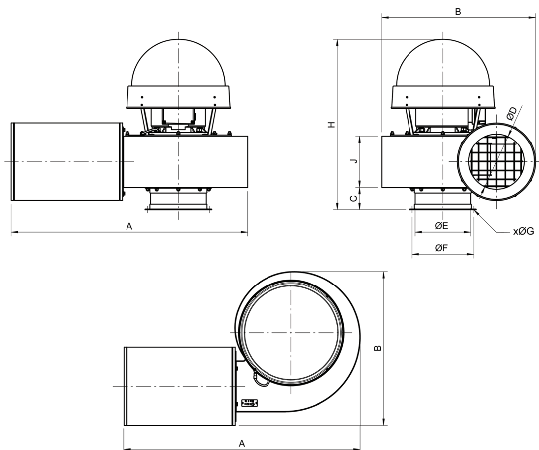
Widok wentylatora od spodu
