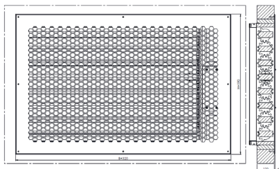
Rysunek 5. Maskownica płaska MKW-B.
