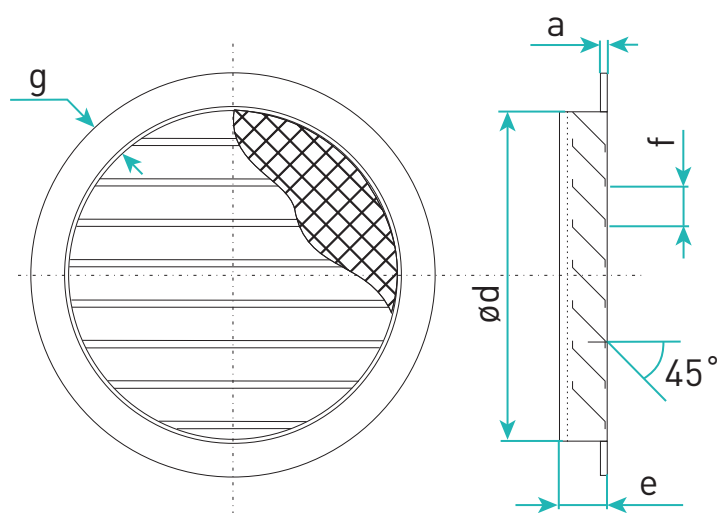
Rysunek 1. Wymiary czerpni CSO.
