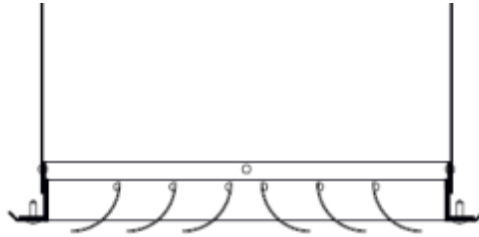
Rysunek 6 Montaż nawiewnika do skrzynki rozprężnej za pomocą bocznych wkrętów
