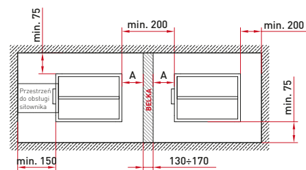
Rysunek 5. Wymagane odległości między klapami montowanymi pojedynczo.
