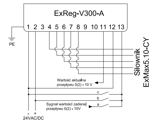
Funkcja A (Menu 7.1: 0/2...10V/12+)
