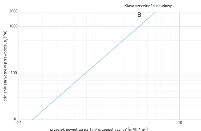
Wykres 3. Przekieki powietrza przez przegrodę przepustnicy PWS (pełne zamknięcie).
