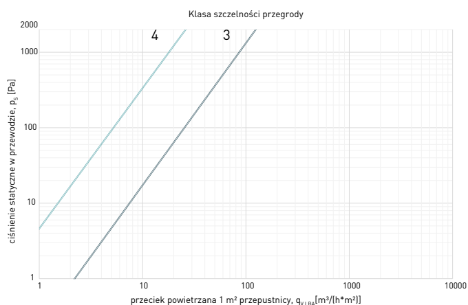
Wykres 2. Przekieki powietrza przez przegrodę przepustnicy PWS (pełne zamknięcie).
