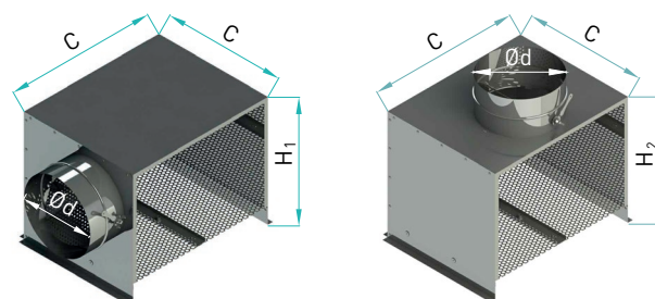
Rysunek 2. Wymiary kwadratowych skrzynek rozprężnych SR do paneli NS5-K.
