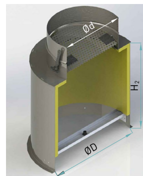
Rysunek 3. Wymiary okrągłych skrzynek rozprężnych SRR do paneli NS5-R.
