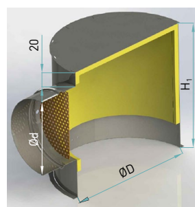
Rysunek 3. Wymiary okrągłych skrzynek rozprężnych SRR do paneli NS5-R.
