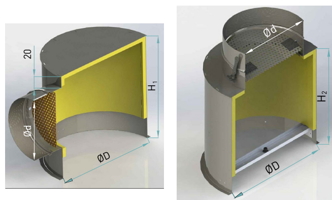
Rysunek 3. Wymiary okrągłych skrzynek rozprężnych SRR do paneli NS8-K.
