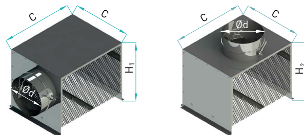
Rysunek 2. Wymiary kwadratowych skrzynek rozprężnych SR do paneli NS8-K.
