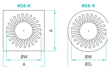
Rysunek 1. Wymiary paneli czołowych NS8.
