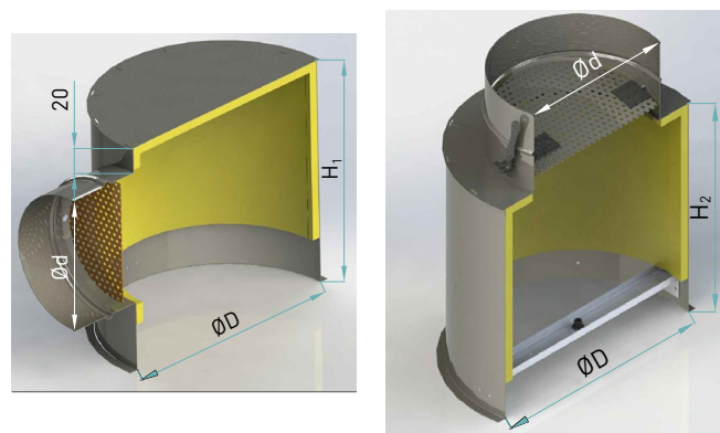
Rysunek 3. Wymiary okrągłych skrzynek rozprężnych SRR do paneli NS9-RR.
