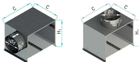
Rysunek 2. Wymiary kwadratowych skrzynek. SR do paneli NS9-KR i NS9-KK.
