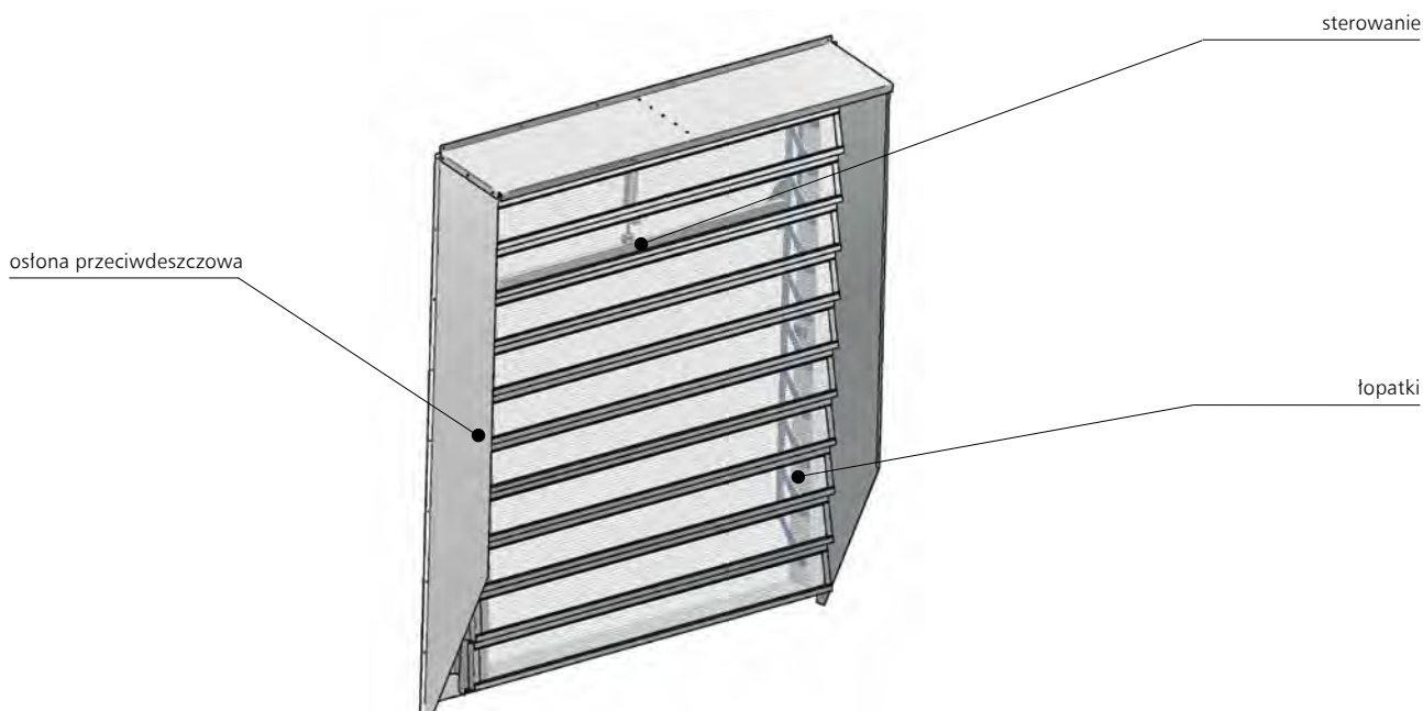
Rys. 176 - Budowa klapy żaluzyjowej napowietrzającej mcr LAM-N wyposażonej w osłonę przeciwdeszczową
