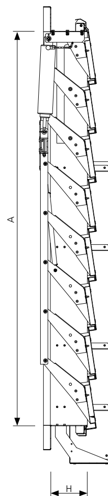
Rys. 175 – Przekrój A-A klapy żaluzjowej oddymiającej mcr LAM w pozycji zamkniętej, (montaż na dachu)
