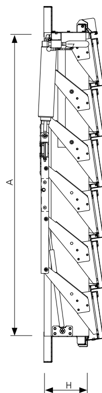
Rys. 179 – Przekrój A-A przez klapę żaluzjową napowietrzającą mcr LAM-N w pozycji zamkniętej, (montaż w fasadzie)
