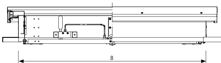
Rys. 177 – Przekrój B-B przez klapę żaluzjową napowietrzającą mcr LAM-N w pozycji zamkniętej (montaż w fasadzie)
