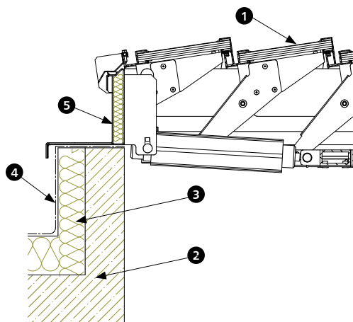
Rys. 180 - Montaż klapy żaluzyjowej z podstawą nakładkową ocieploną na dachu, na istniejącym cokole
