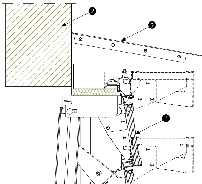
Rys. 186 - Montaż kłapy żaluzyjowej bezpośrednio do ściany (fasady) od strony zewnętrznej
