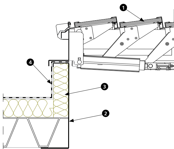
Rys. 181 - Montaż klapy żaluzyjowej z podstawą nakładkową nieocieploną na dachu, na cokole stalowym
