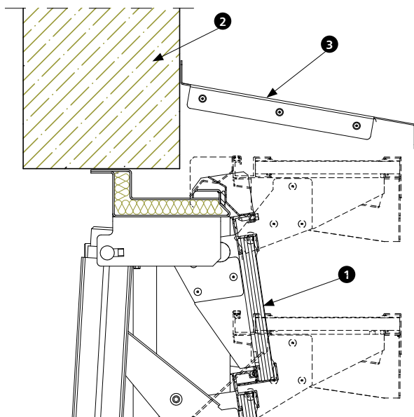
Rys. 185 - Montaż kłapy żaluzyjowej bezpośrednio do ściany (fasady)
