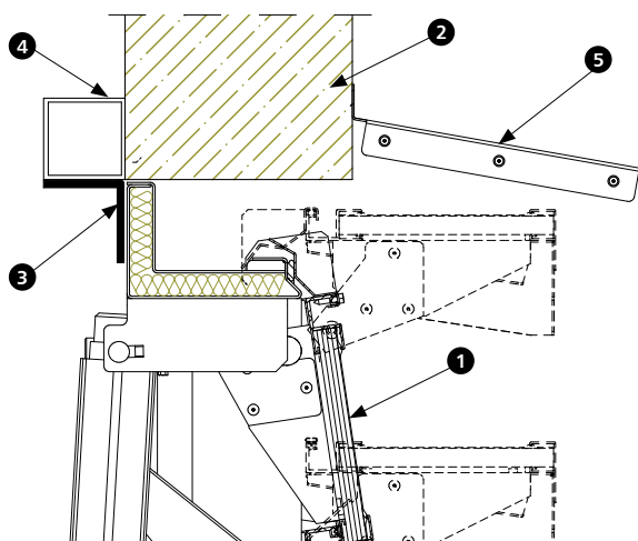
Rys. 183 - Montaż kłapy żaluzyjowej w ścianie (fasadzie) za pomocą dodatkowego profilu stalowego
