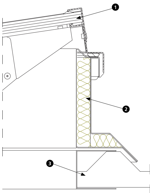
Rys. 182 - Montaż klapy żaluzyjowej na dachu systemowym krytym blachą
