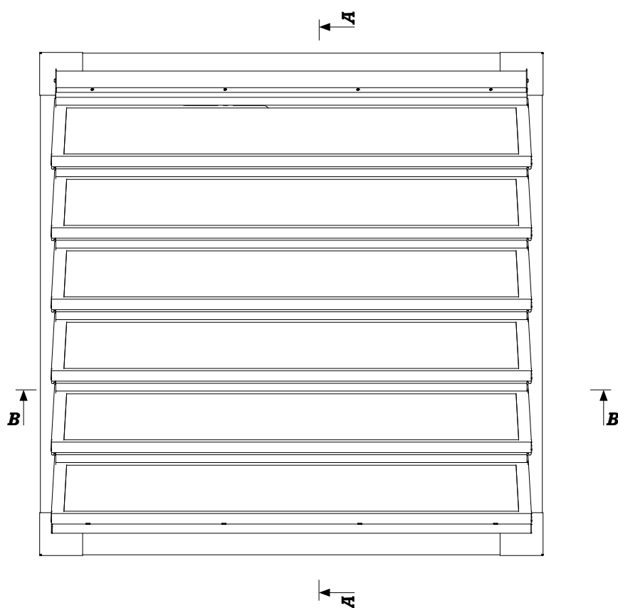
Rys. 178 – Widok z góry klapy żaluzjowej napowietrzającej mcr LAM-N w pozycji zamkniętej
