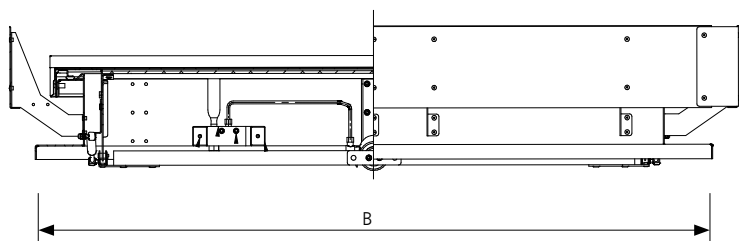
Rys. 173 – Przekrój B-B przez klapę żaluzjową oddymiającą mcr LAM w pozycji zamkniętej (montaż na dachu)
