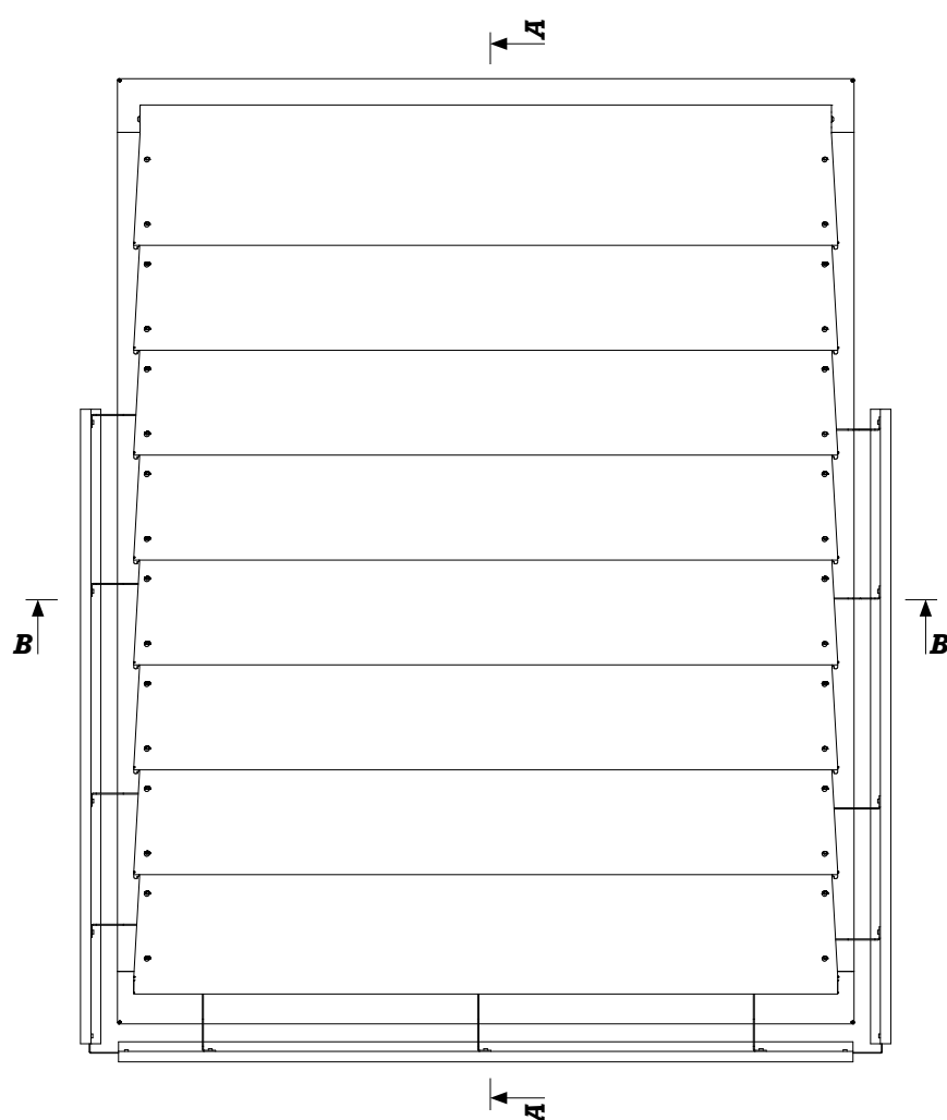
Rys. 174 – Widok z góry klapy oddymiającej żaluzjowej mcr LAM w pozycji zamkniętej
