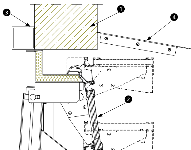
Rys. 184 - Montaż kłapy żaluzyjowej w ścianie (fasadzie) do konstrukcji wsporczej
