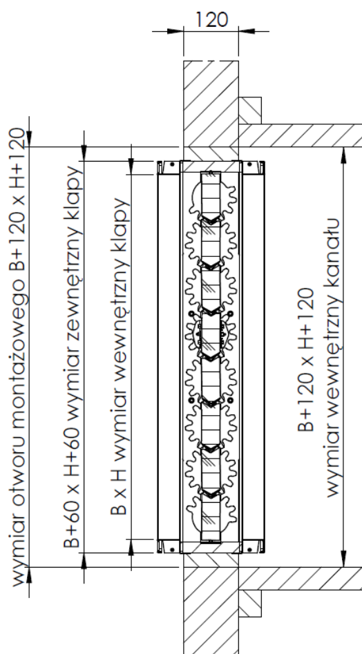
Rys. 4. Sposób zabudowy klap odcinających WKP-P z kanałem z płytą PROMAT
