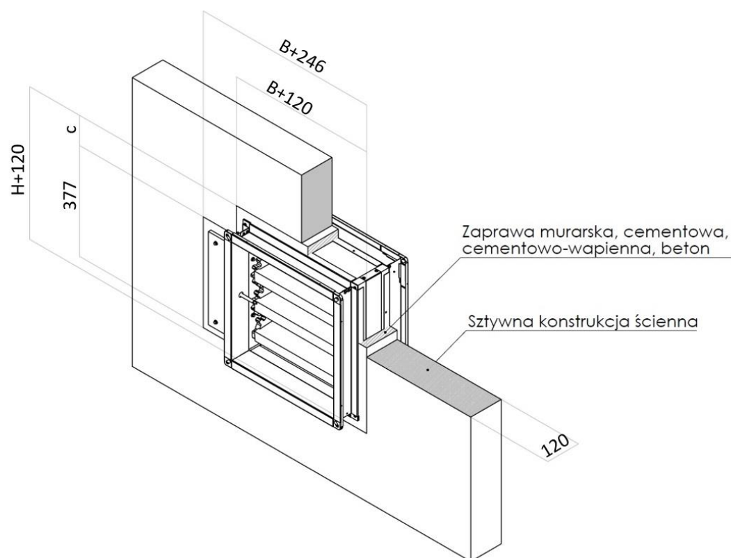
Rys. 1. Wymiary otworu montażowego klap odcinających WKP-P w sztywnych konstrukcjach ściennych z poziomą i pionową osią obrotu przegrody.
