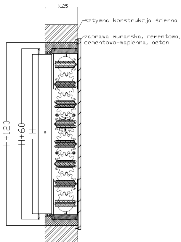
Rys. 5. Sposób zabudowy klapy odcinającej WKP-P w konstrukcjach o grubości większej niż 125 mm
