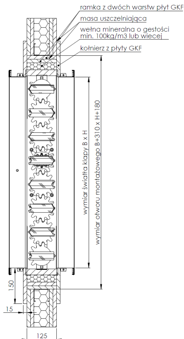
Rys. 6. Sposób zabudowy kłap WKP-P w podatnych konstrukcjach ściennych o grubości 125 mm
