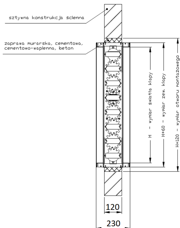
Rys. 2. Sposób zabudowy klap odcinających WKP-P w sztywnych konstrukcjach ściennych. Oś przegrody powinna się pokrywać z osią ściany.
