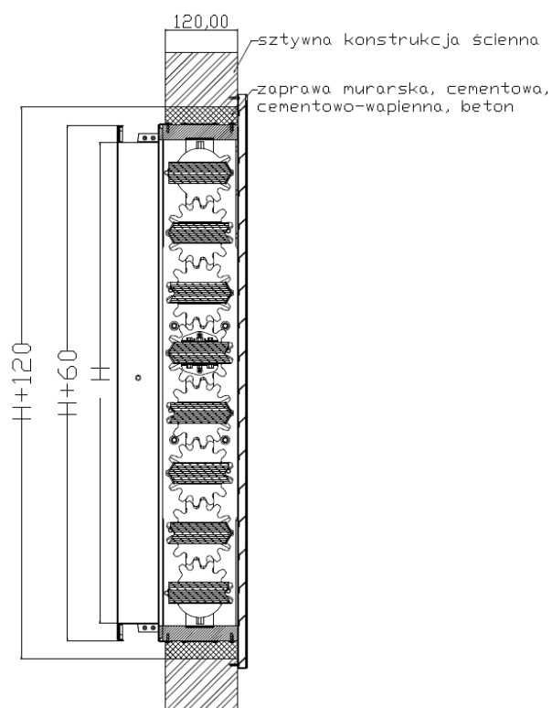
Rys. 3. Sposób zabudowy klap odcinających WKP-P z kratką KST w sztywnych konstrukcjach ściennych.
