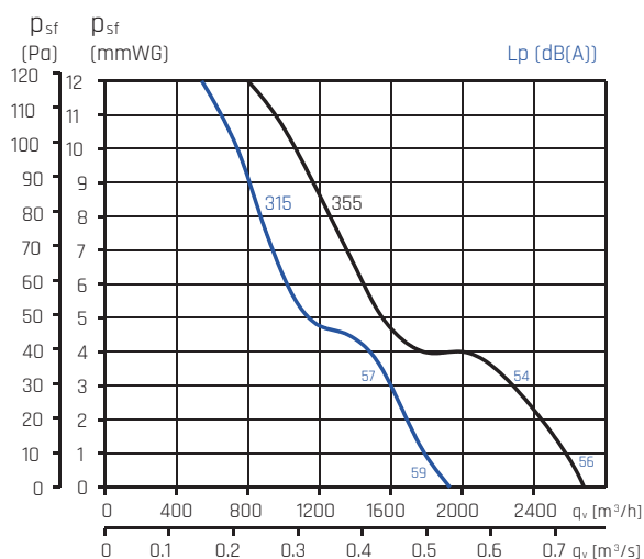
315-355 4-biegunowe
