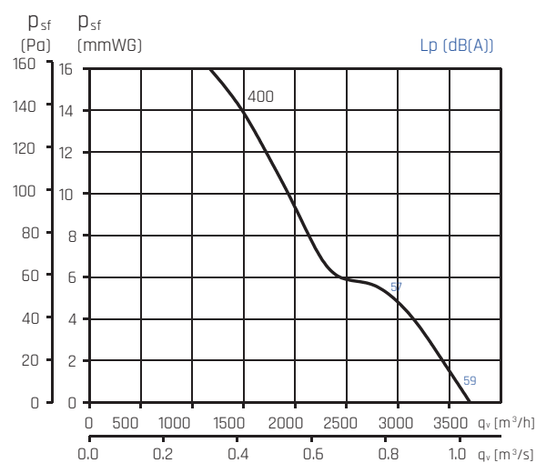
400 4-biegunowe
