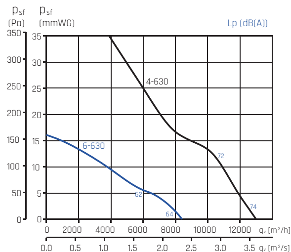
630 4- i 6-biegunowe
