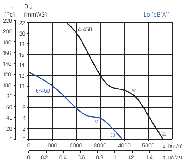
450 4- i 6-biegunowe
