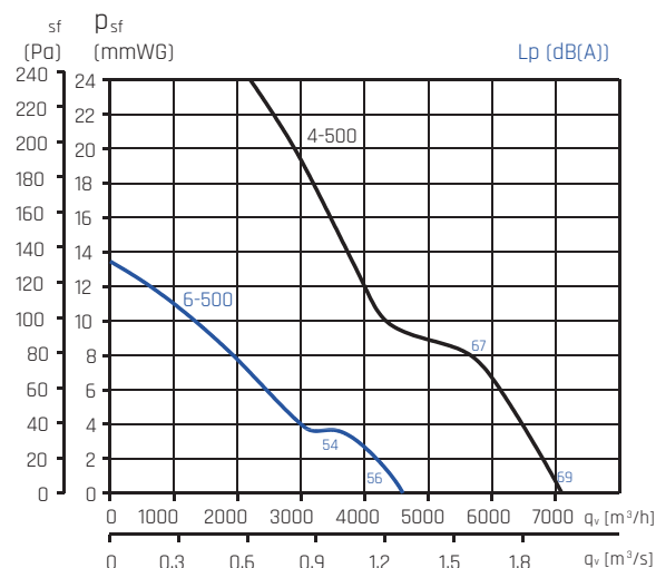
500 4- i 6-biegunowe
