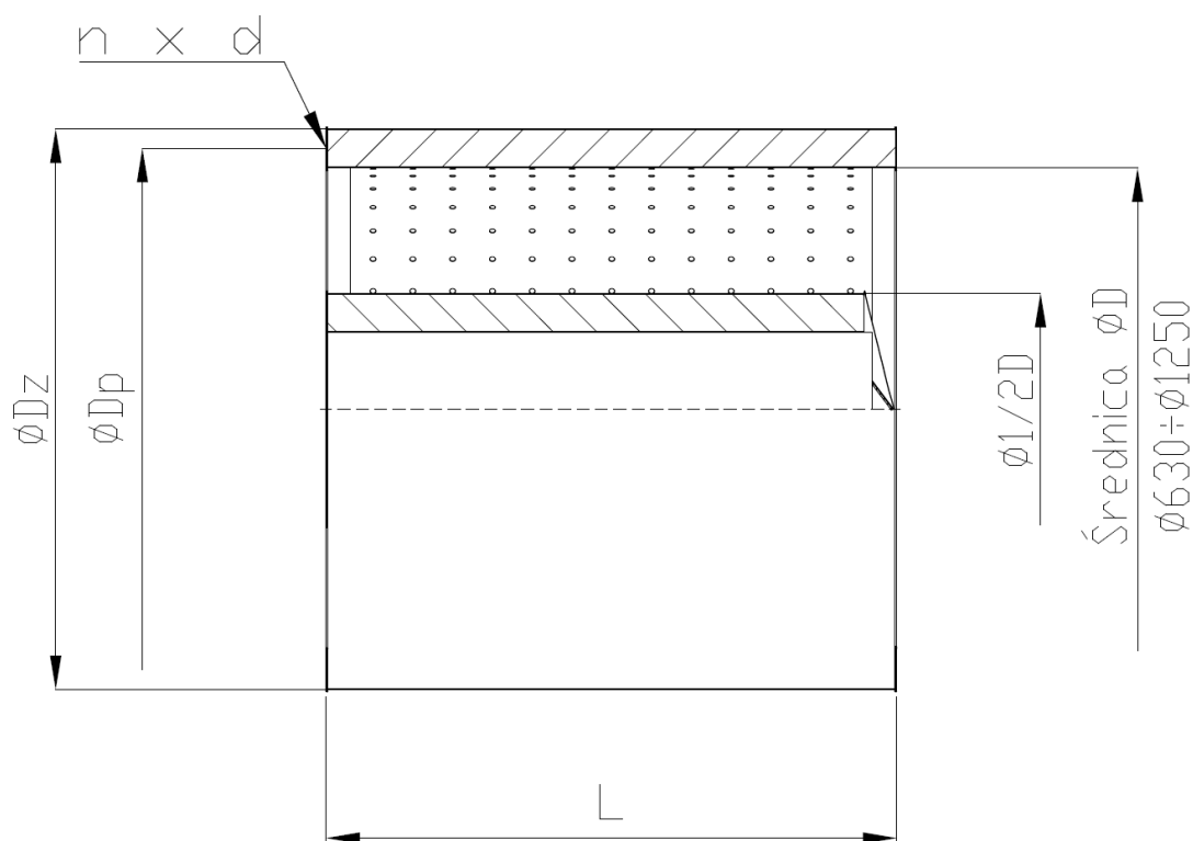
Rys. 8. Zasady wymiarowania tłumików TL-CN
