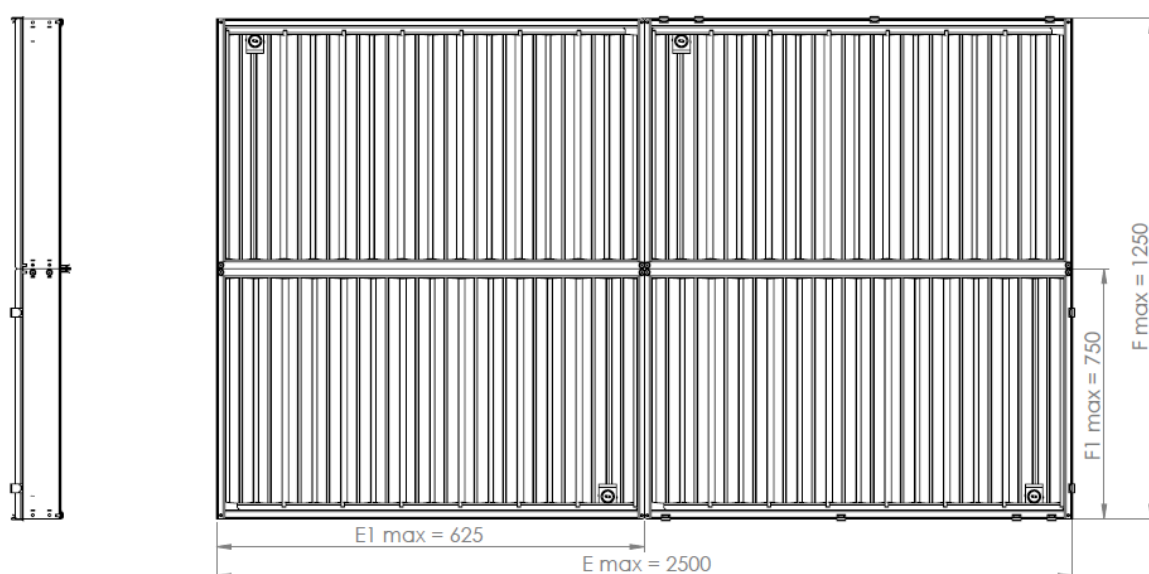
Rys. 14. Zasady wymiarowania przepustnic SDS-GP
