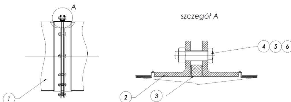
Rys.16. Szczegół połączeń elementów kołowych
