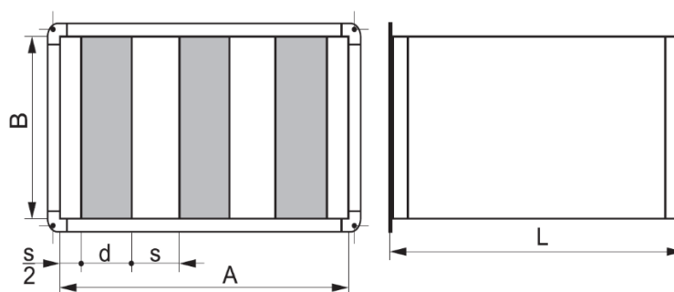
Rys. 6. Zasady wymiarowania tłumików TAP
