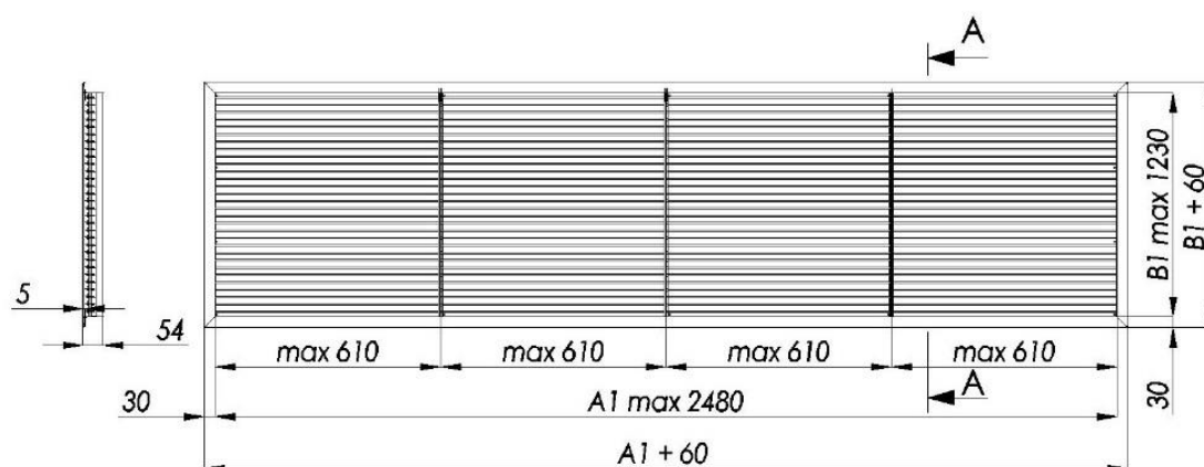
Rys. 11. Zasady wymiarowania kratki SDS-STW
