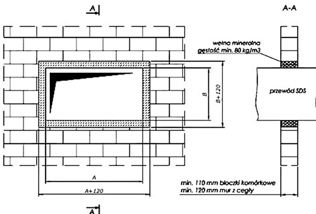
Rys. 19. Szczegóły przejścia instalacji SDS przez pionową przegrodę budowlaną
