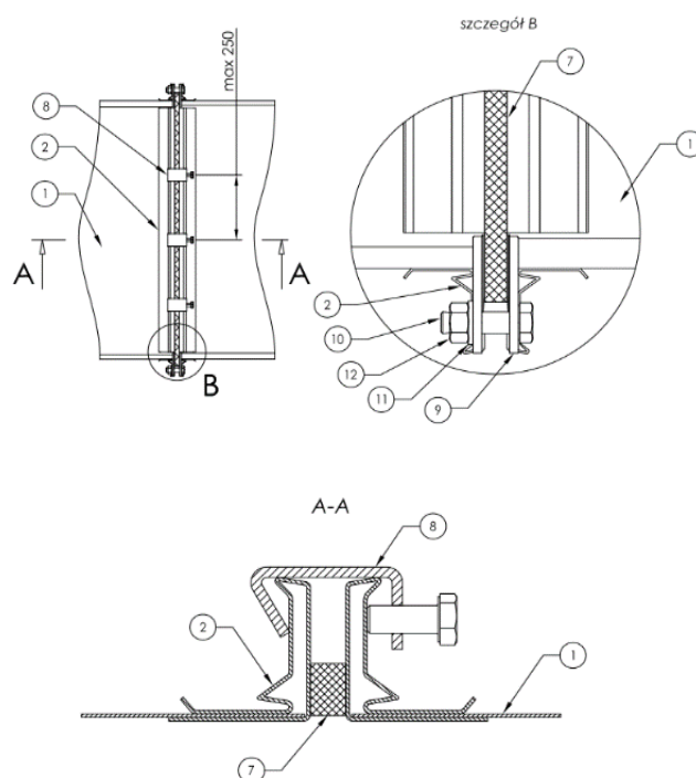
Rys.15. Szczegóły połączeń kołnierzowych elementów prostokątnych
