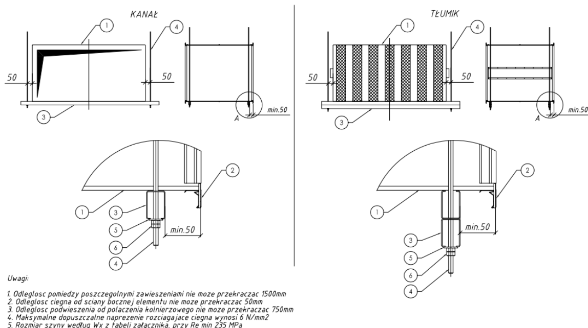
Rys. 17. Szczegóły montażowe instalacji typu SDS
