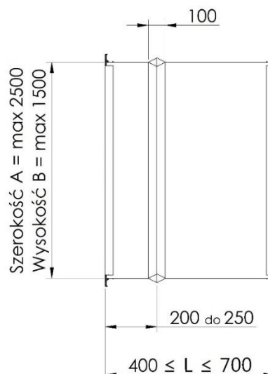
Rys. 2. Zasady wymiarowania kanałów kompensacyjnych SDS-DC
