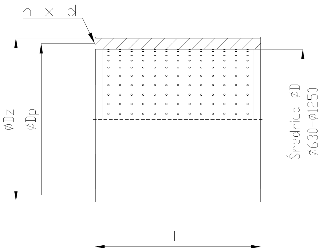
Rys.9. Zasady wymiarowania tłumików TL-C
