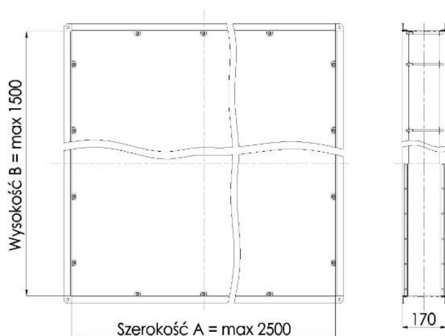
Rys. 3. Zasady wymiarowania kompensatorów SDS-KE
