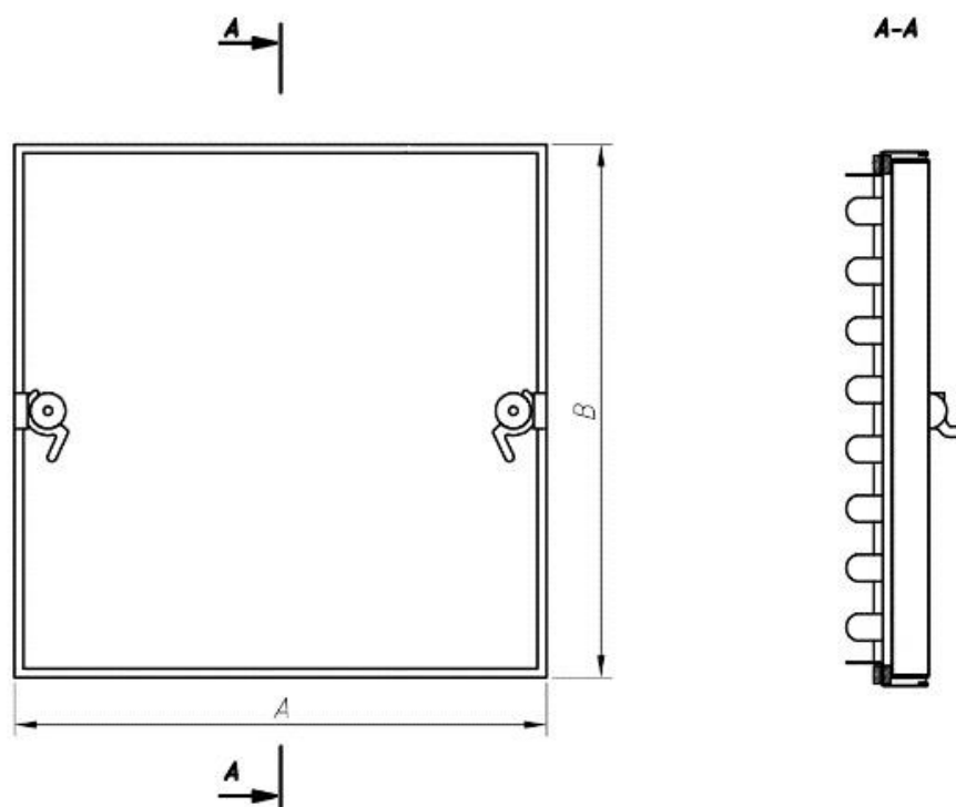
Rys. 10. Zasady wymiarowania włazów rewizyjnych
