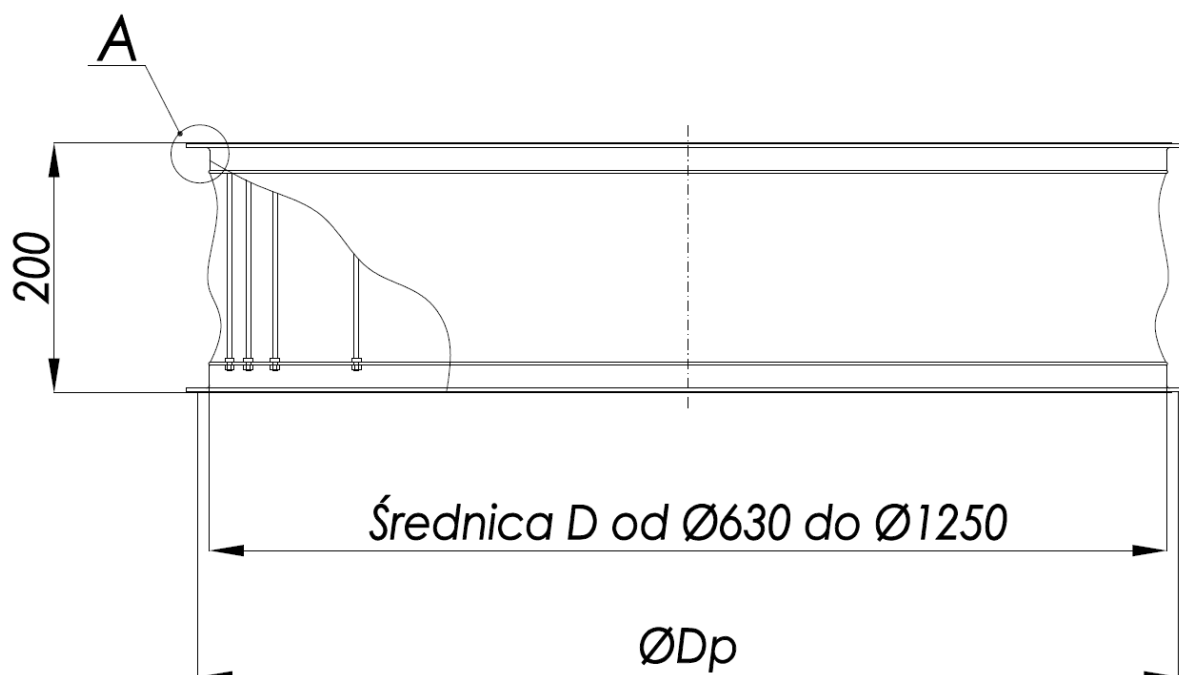
Rys. 4. Zasady wymiarowania kompensatorów
