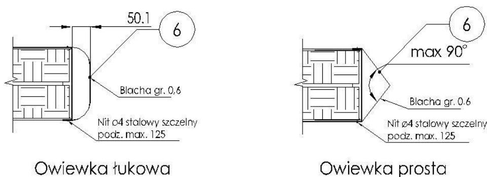
Rys. 7. Budowa owiewek tłumików TAP
