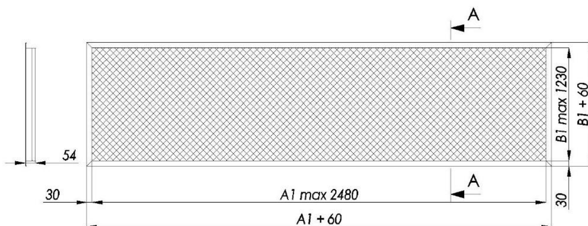
Rys. 12. Zasady wymiarowania kratki SDS-STW
