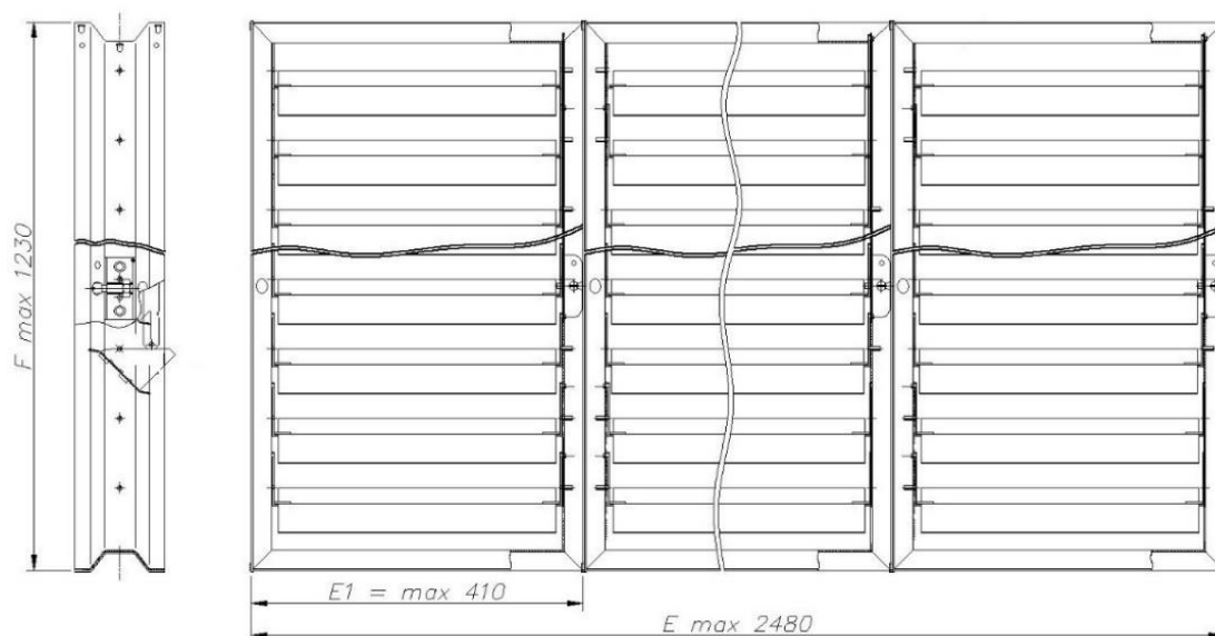
Rys. 13. Zasady wymiarowania przepustnic SDS-GS
