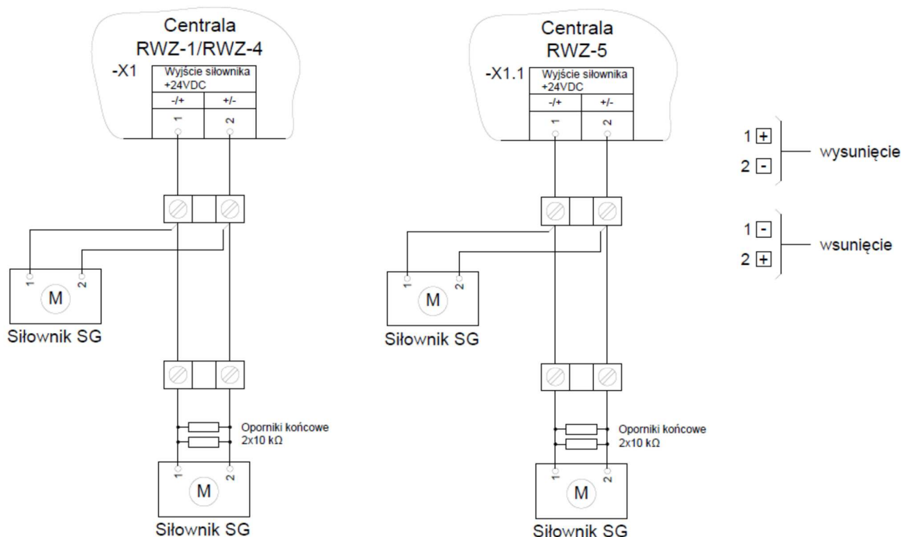
Rys. 47. Schematy podłączenia siłowników do centrali RWZ 5 W centrali RWZ-5 kolejne siłowniki podłączać do zacisków: X1.2, X1.3, X1.4 w zależności od konfiguracji stref dymowych i stref przewietrzania.
