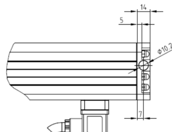
Montaż na dolnym końcu z otworem Ø10,2
