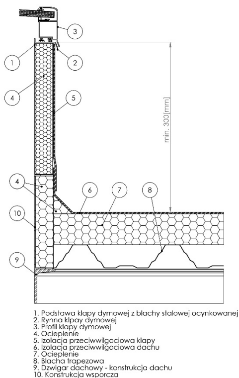
Rys. 63. Montaż kłapy SCD na izolowanym cokole stalowym, z podkonstrukcją nad izolacją.
