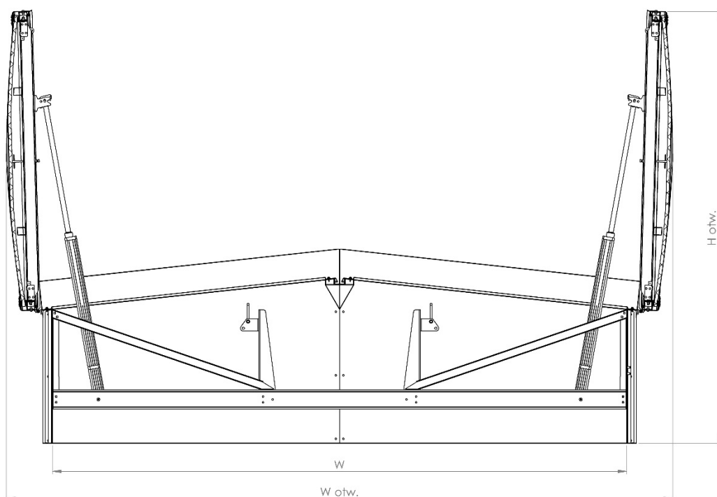
Rys. 6. Kłapa dwuskrzydłowa SCD-2-P... w pozycji otwartej
