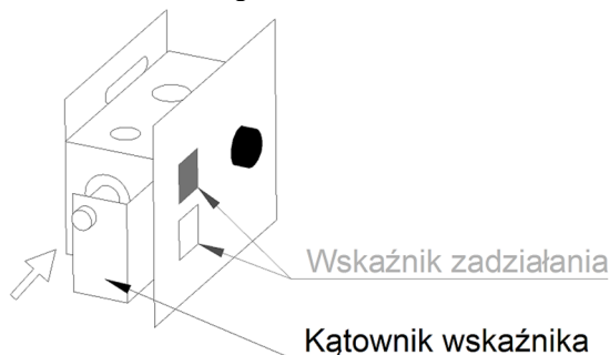
Rys. 28. Uzbrajanie skrzynki AK nabojem CO 2 .
