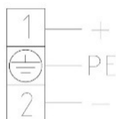
Rys. 30. Schemat podłączenia elektromagnesu.
