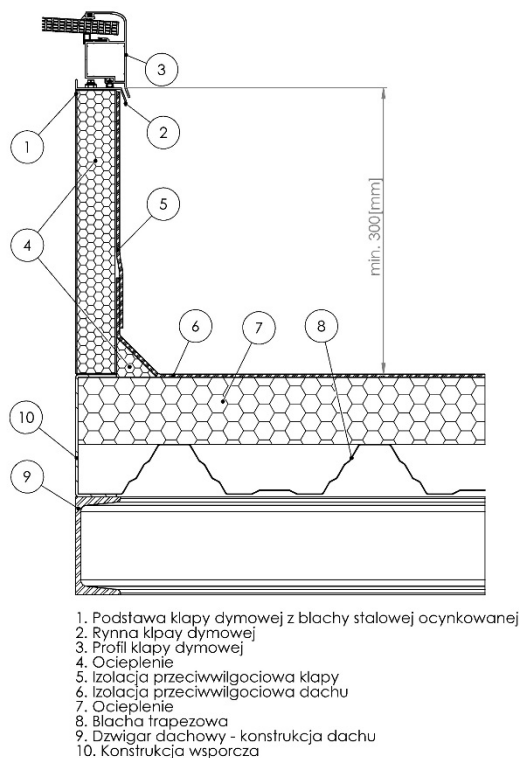
Rys. 59. Montaż kłapy SCD na izolowanym dachu stalowym, bez podkonstrukcji, pod blachą trapezową.
