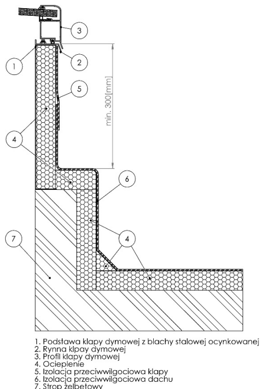
Rys. 64. Montaż kłapy SCD na cokole żelbetonowym.
