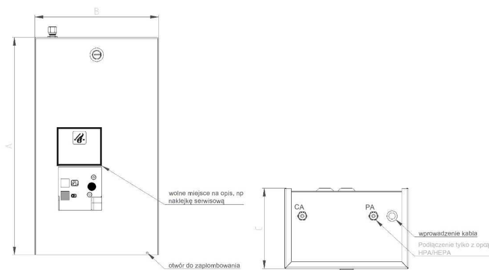
Rys. 26. Wymiary skrzynek alarmowych.
