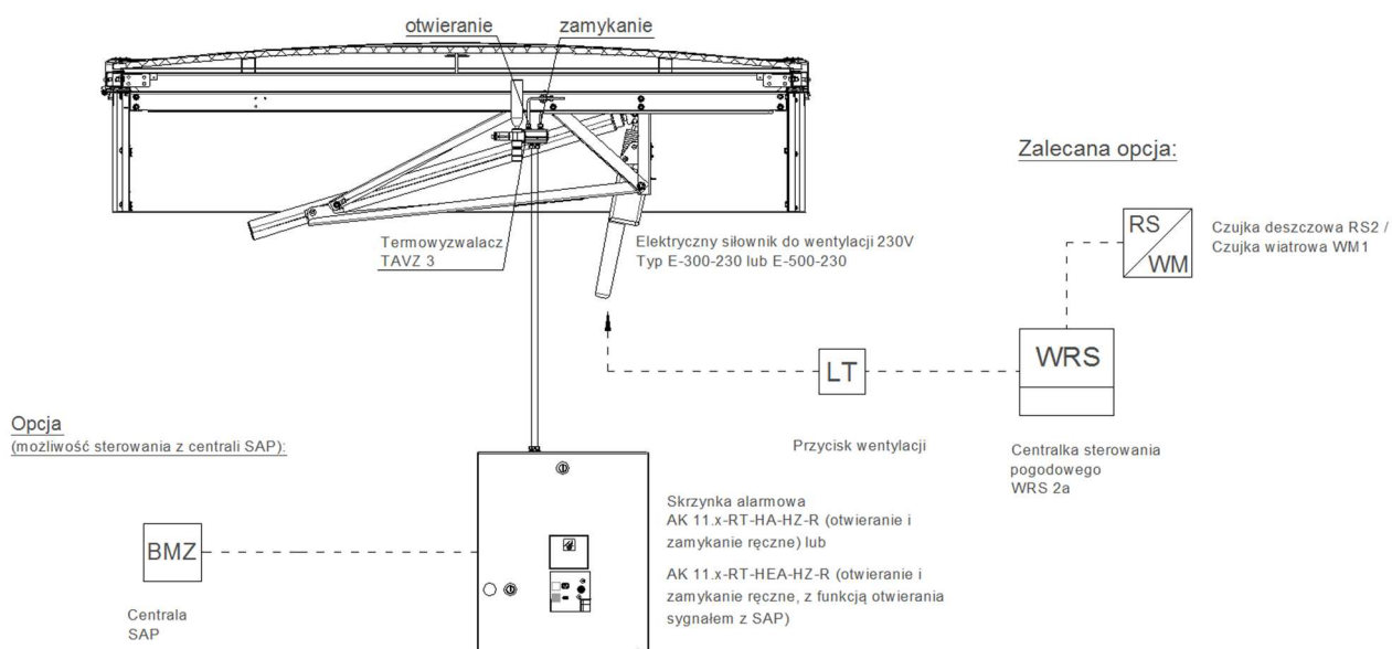
Rys. 15. Kłapa typ „B” z siłownikiem pneumatycznym, termowyzwalaczem, skrzynką alarmową. Otwieranie ręczne lub automatyczne po przekroczeniu temperatury, lub sygnałem z SAP (z modułem elektrycznym w skrzynce AK). Wentylacja za pomocą siłownika elektrycznego.
