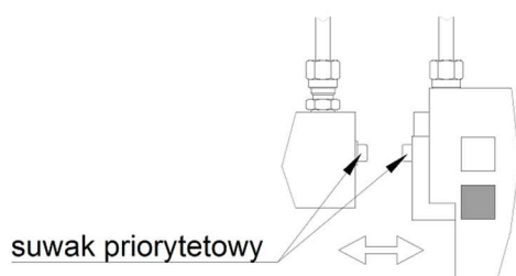
Rys. 29. Uzbrajanie skrzynki AK nabojem CO 2 .
