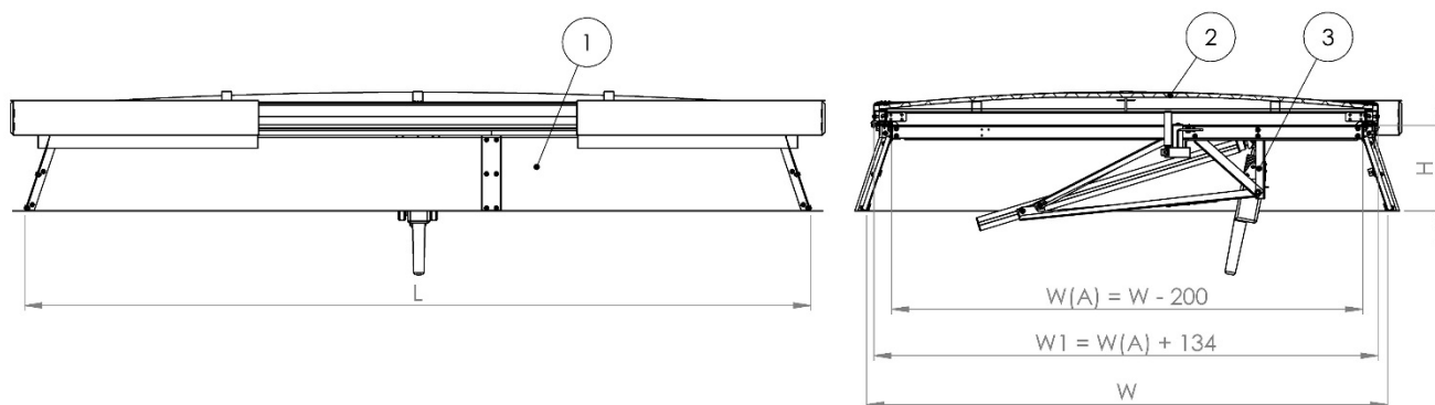
Rys. 1. Kłapa jednoskrzydłowa na podstawie prostej SCD-1-P...
