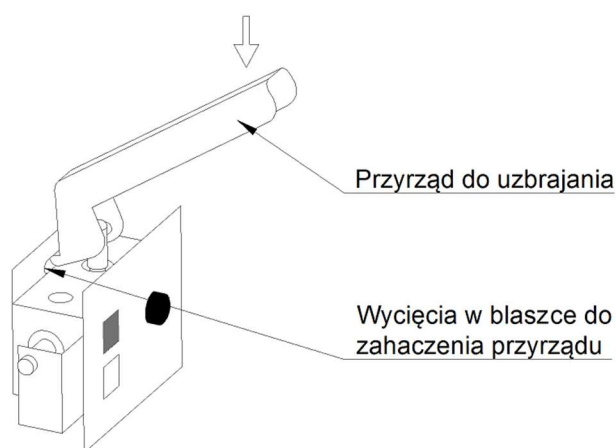
Rys. 27. Uzbrajanie skrzynki AK nabojem CO 2 .
