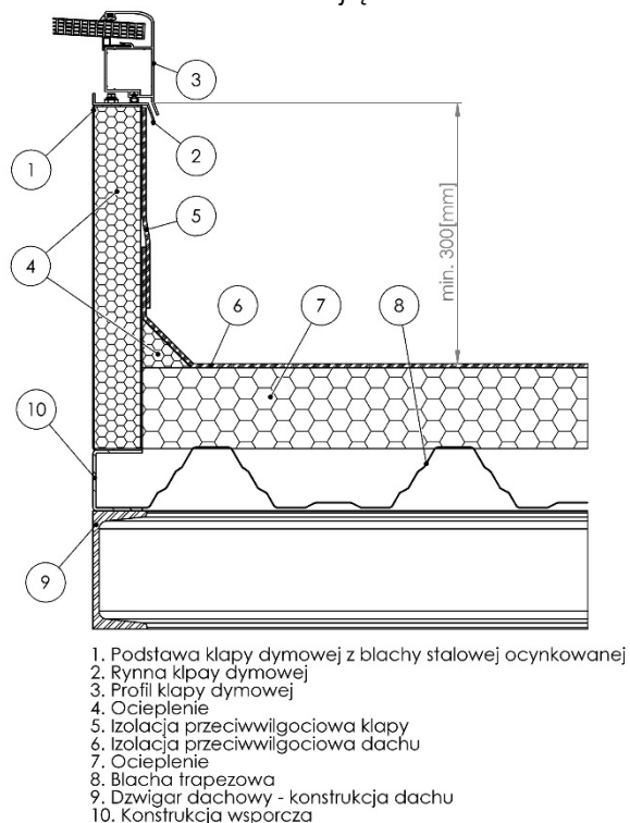
Rys. 62. Montaż kłapy SCD na izolowanym dachu stalowym, z podkonstrukcją, nad izolacją.
