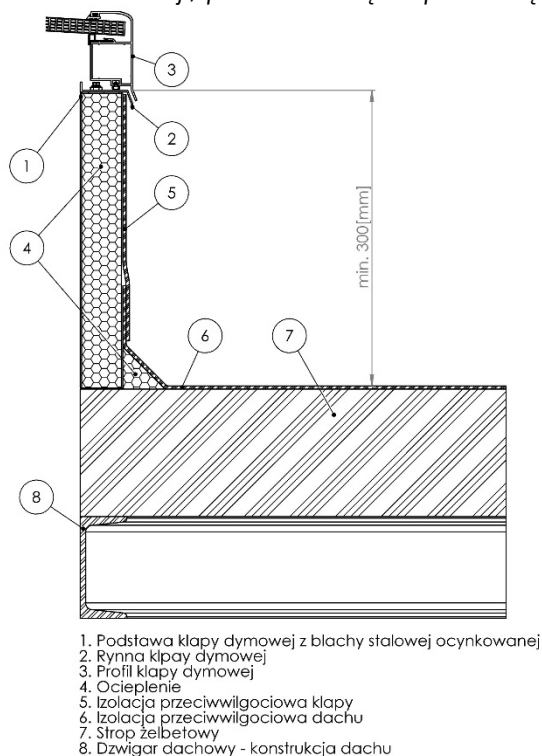
Rys. 61. Montaż kłapy SCD na dachu żelbetonowym.
