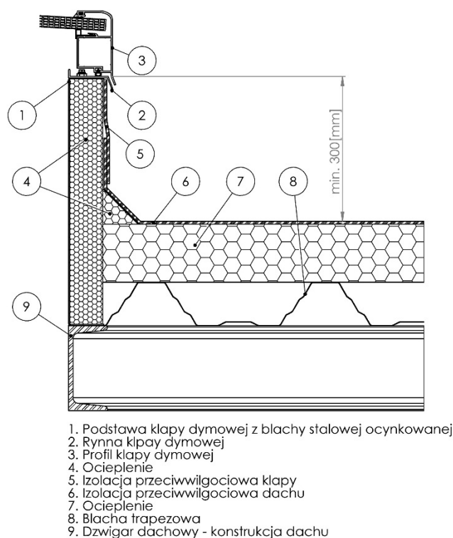
Rys. 60. Montaż kłapy SCD na izolowanym dachu stalowym, z podkonstrukcją, pod izolacją.
