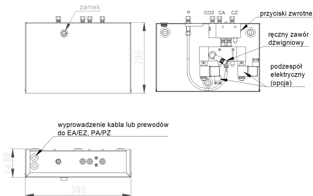
Rys. 32. Wymiary skrzynek PLZ.
