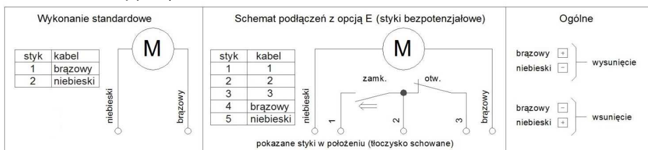
Rys. 42. Schemat podłączeń.
