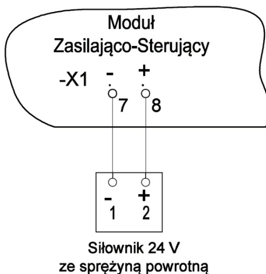
Rysunek 5.80. Schemat podłączenia przepustnicy SRC
