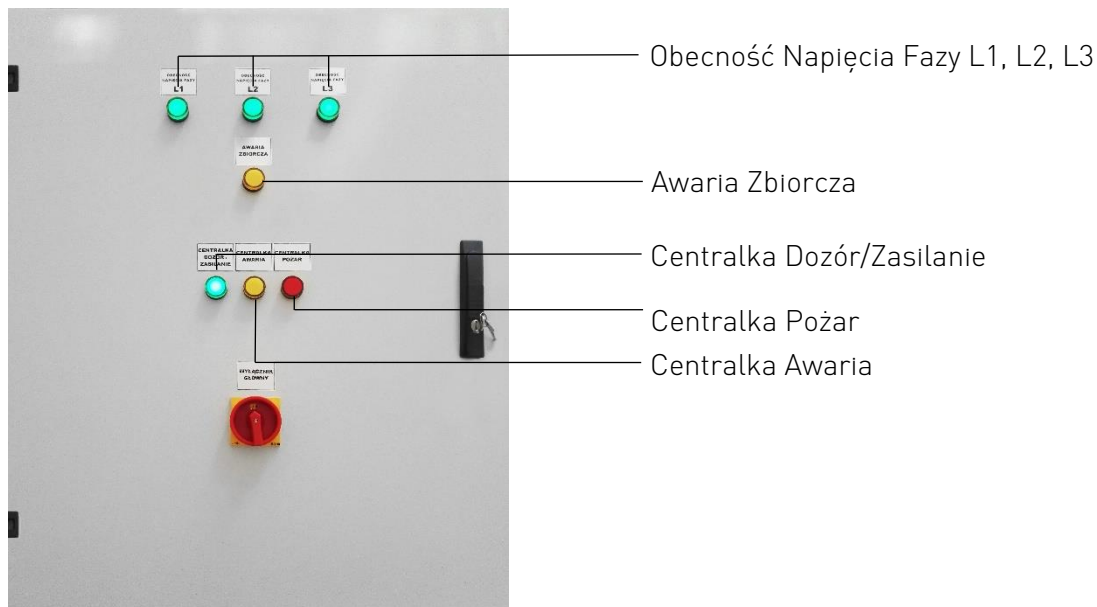
Rysunek 7.1. Diody sygnalizacyjne na froncie MZS
