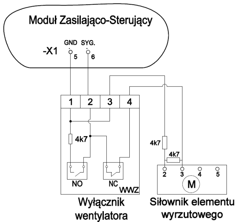
Rysunek 5.70. Schemat podłączenia krańcówek siłownika klapy oraz wyłącznika wentylatora
