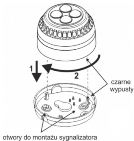
Rysunek 6.19. Schemat zamykania sygnalizatora i rozmieszczenie otworów montażowych
