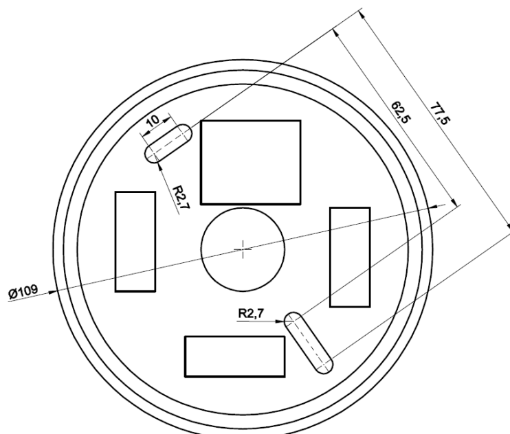
Rysunek 5.13. Wymiary i rozmieszczenie otworów montażowych gniazda czujki CDZ-2
