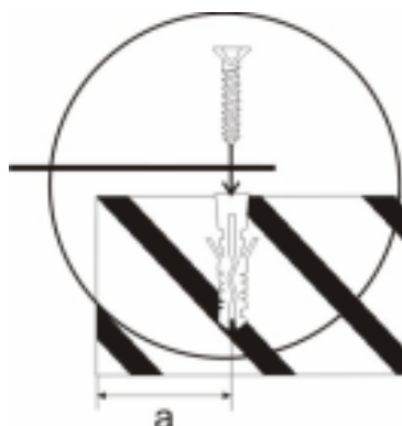
Rysunek 5.47. Ilustracja wytycznych posadowienia kłapy SCD-1-L na konstrukcji dachu
