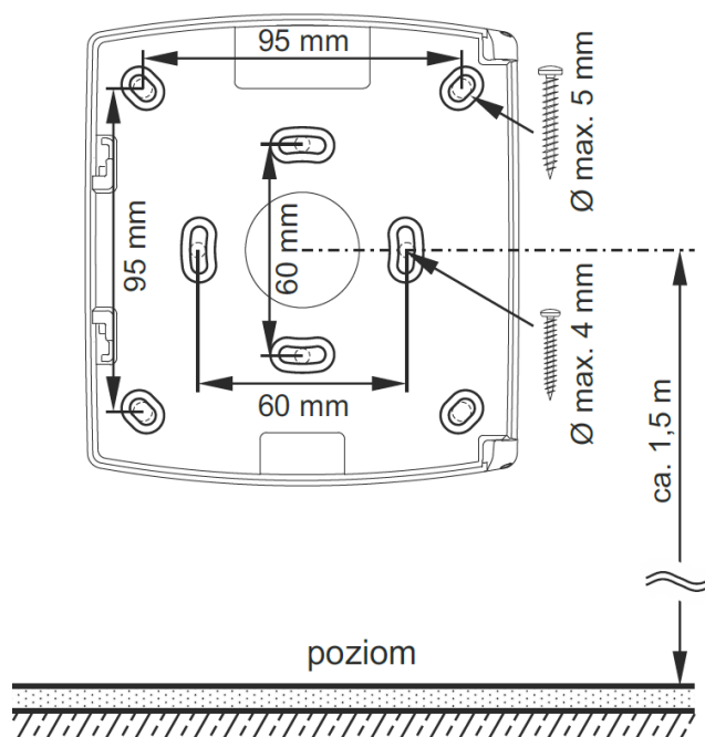
Rysunek 5.36. Wymiary i rozmieszczenie otworów montażowych przycisków POZ-4, POZ-5, POZ-6
