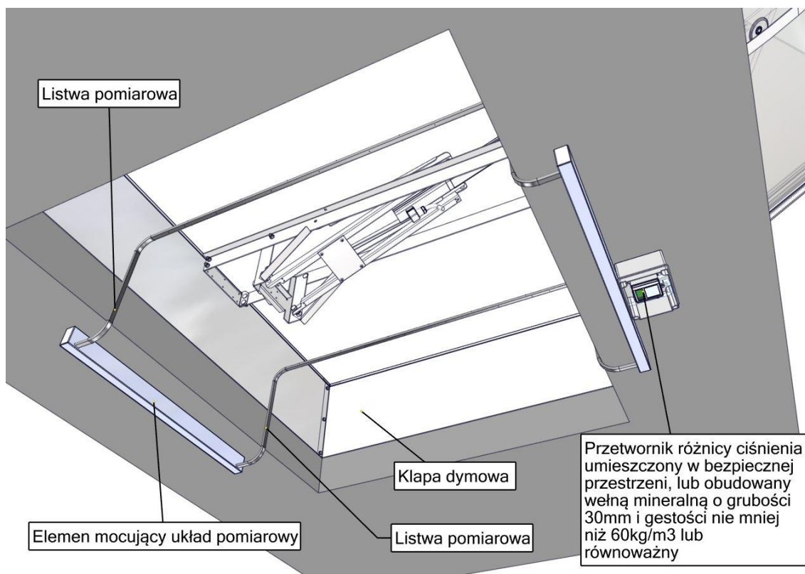
Rysunek 5.84. UPZ w otworze klapy dymowej
