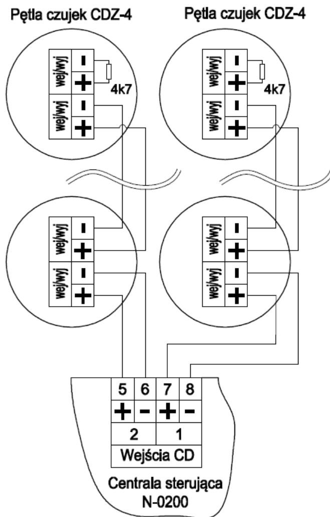
Rysunek 5.17. Schemat podłączenia czujek dymu CDZ-4
