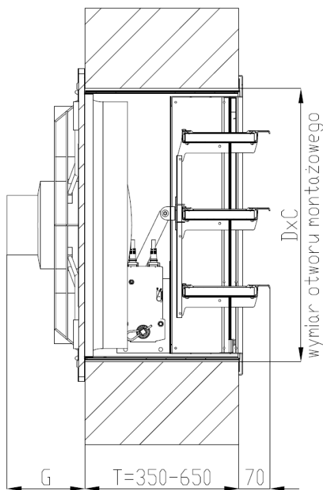
Rysunek 5.74. Zabudowa ZNZ
