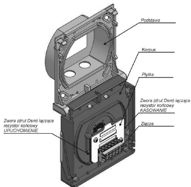
Rysunek 5.24. Przycisk po otwarciu
