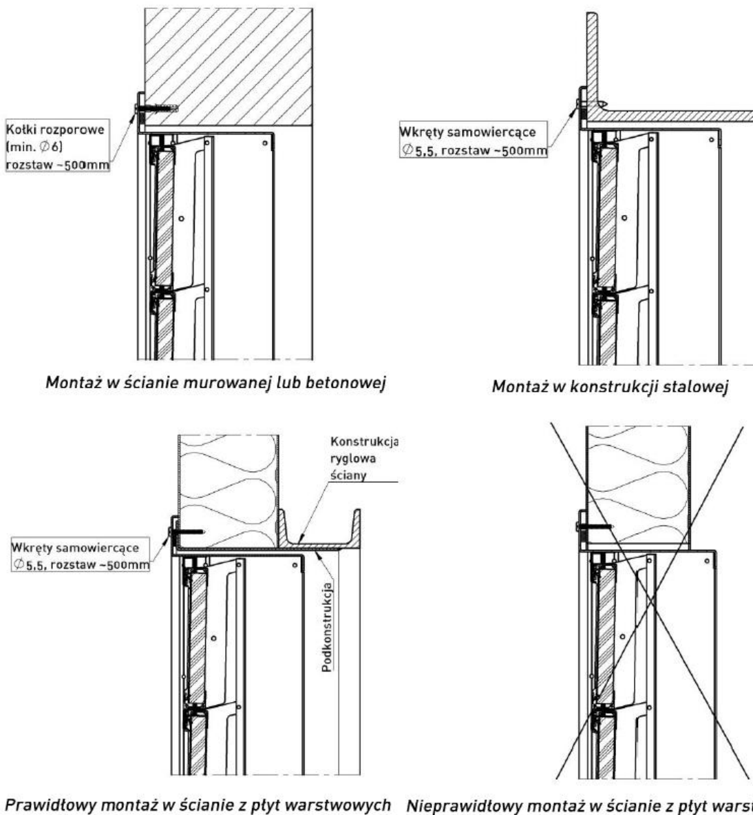
Rysunek 5.63. Przykłady montażu czerpni CDH-K
