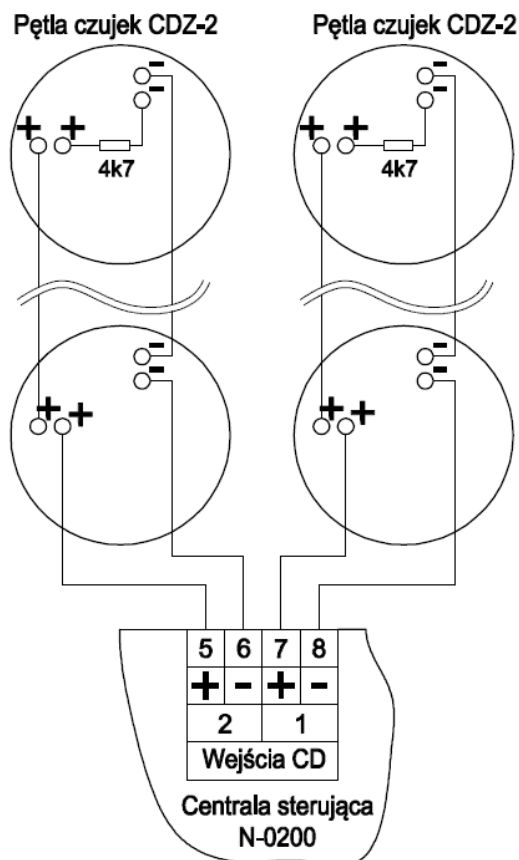
Rysunek 5.12. Schemat podłączenia czujek dymu CDZ-2
