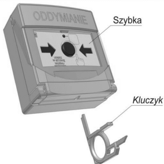
Rysunek 5.21. Wybicie wciśniętego przycisku pożar i zwolnienie blokady szybki
