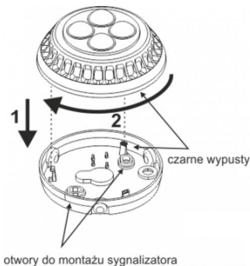
Rysunek 6.16. Schemat zamykania sygnalizatora i rozmieszczenie otworów montażowych
