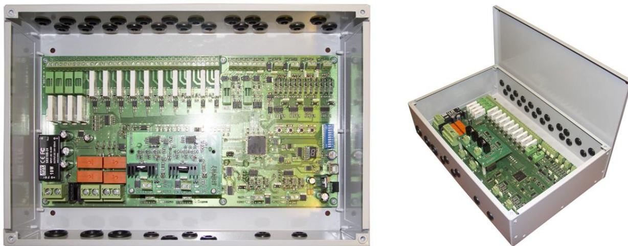
Rysunek 5.3. Część Sterująca Modułu Zasilająco-Sterującego
