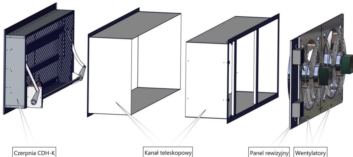
Rysunek 5.73. Zespół napowietrzający ZNZ – elementy składowe.
