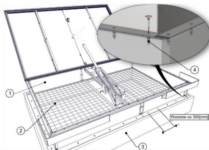
Rysunek 5.50. Montaż kraty przeciwupadkowej KZU
