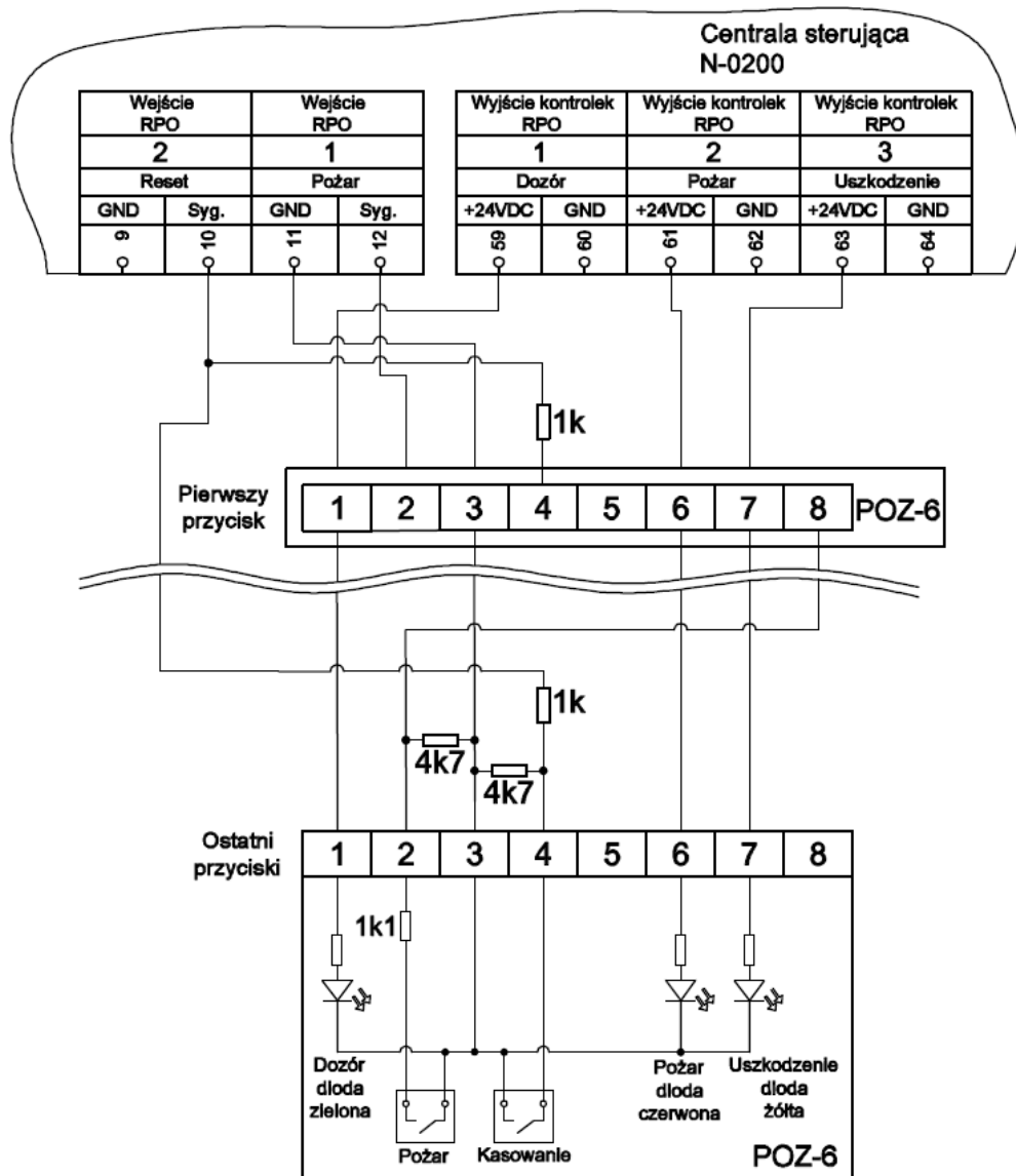
Rysunek 5.34. Schemat podłączenia przycisku POZ-4, POZ-5, POZ-6
