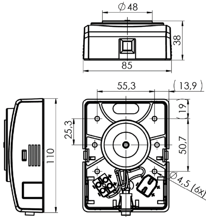
Rysunek 6.22. Wymiary i rozmieszczenie otworów montażowych elektrotrzymacza uniwersalnego
