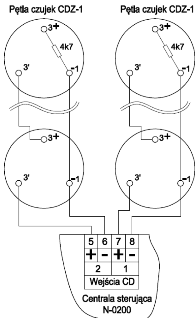
Rysunek 5.10. Schemat podłączenia czujek dymu CDZ-1
