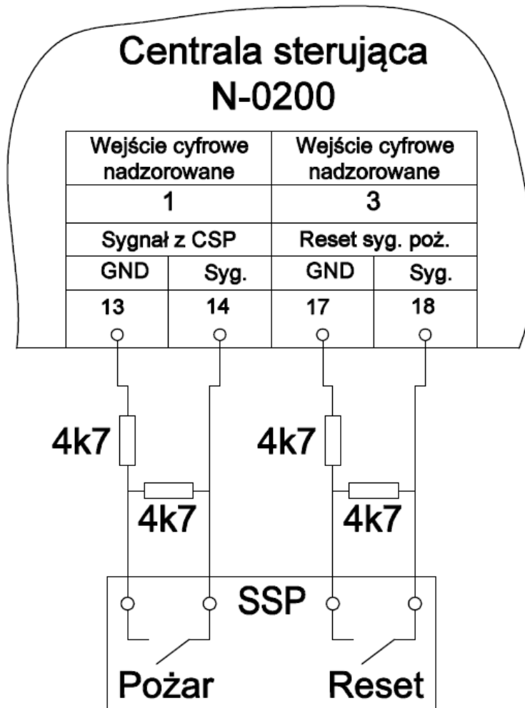
Rysunek 6.29. Schemat podłączenia SSP
