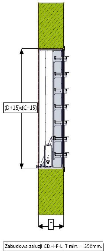
Rysunek 5.83. Zabudowa wyrzutni CDH-F-L
