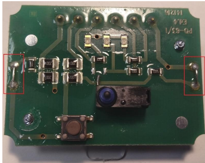
Rysunek 5.25. Zwory rezystora końcowego linii (druć DSM)
