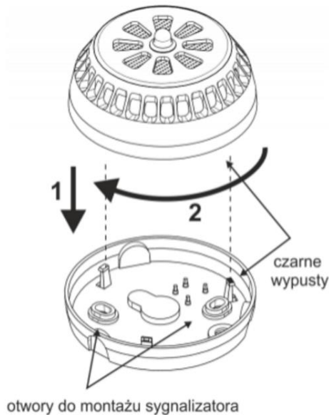
Rysunek 6.13. Schemat zamykania sygnalizatora i rozmieszczenie otworów montażowych
