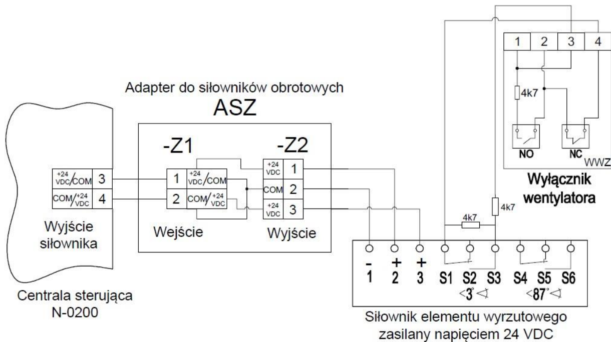
Rysunek 5.82. Schemat podłączenia siłownika Czerpni CDH-F-L
