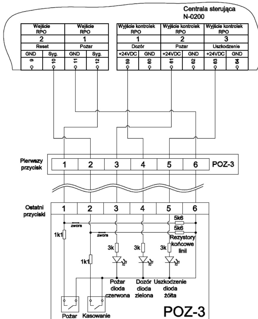
Rysunek 5.28. Schemat podłączenia przycisku POZ-3
