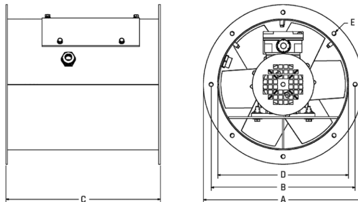
Rysunek 5.68. Wymiary wentylatorów nawiewnych AFC
