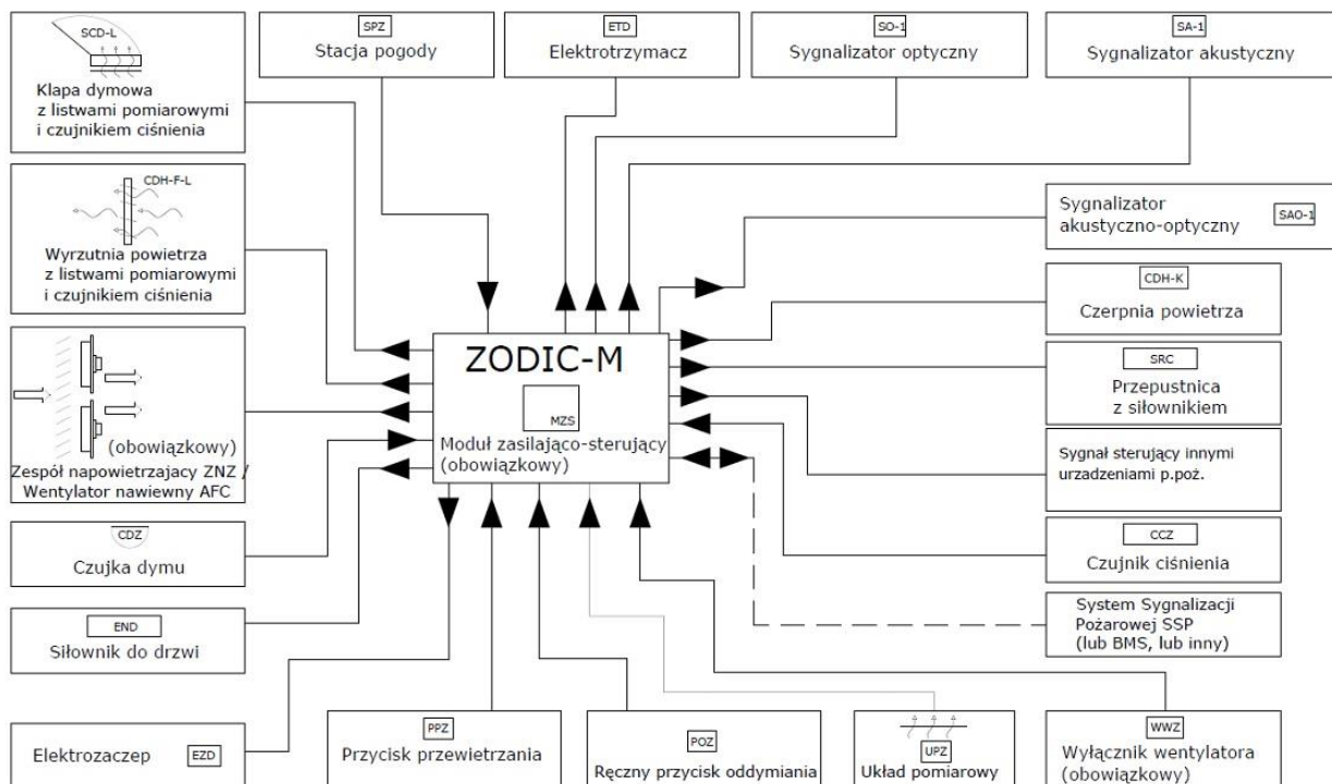
Rysunek 4.1. Schemat ideowy ZODIC-M
