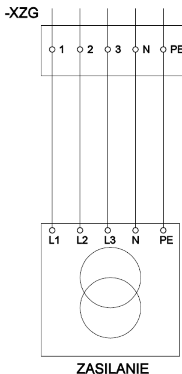
Rysunek 5.8. Schemat podłączenia zasilania do MZS
