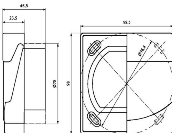
Rysunek 5.30. Wymiary i rozmieszczenie otworów montażowych przycisków POZ-1, POZ-2, POZ-3
