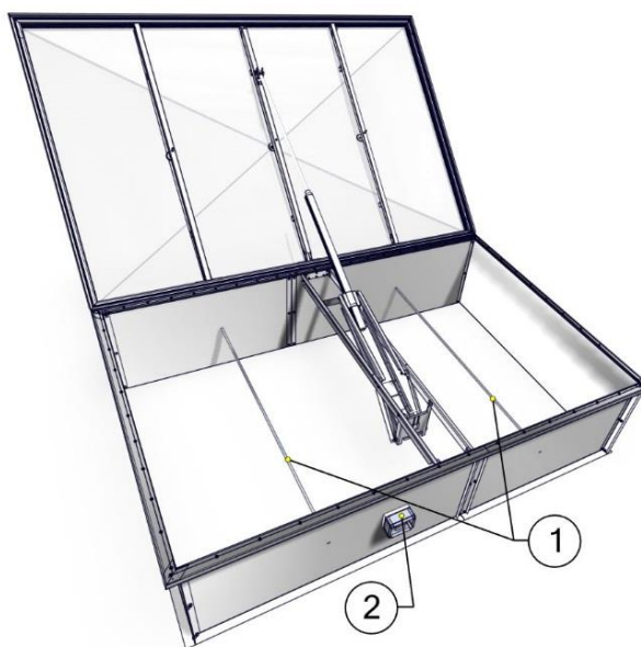
Rysunek 5.38. . Listwy pomiarowe w kłapie SCD-1-L
