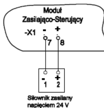
Rysunek 5.75. Schemat podłączenia ZNZ. Po lewej stronie wersja podłączenia wentylatora do zacisków śrubowych, po prawej bezpośrednio do przetwornicy częstotliwości.
