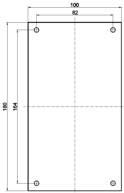
Rysunek 5.71. Wymiary i rozmieszczenie otworów montażowych wyłącznika wentylatora WWZ
