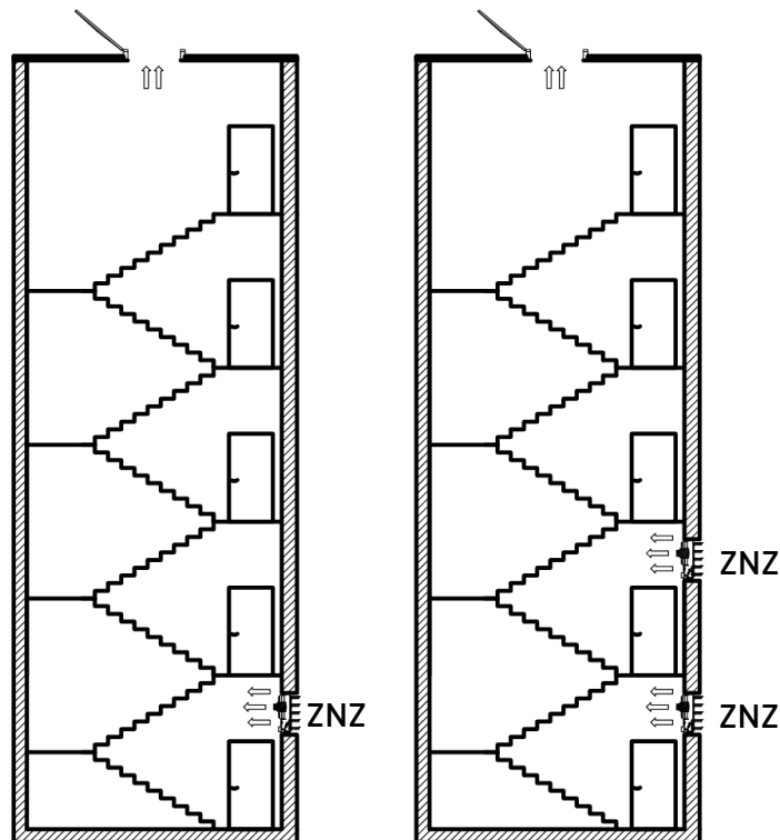
Rysunek 5.76. Przykład z jednym punktem napowietrzającym i z dwoma punktami napowietrzającymi.
