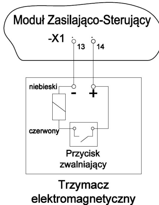
Rysunek 6.21. Schemat podłączenia elektroztrzymacza
