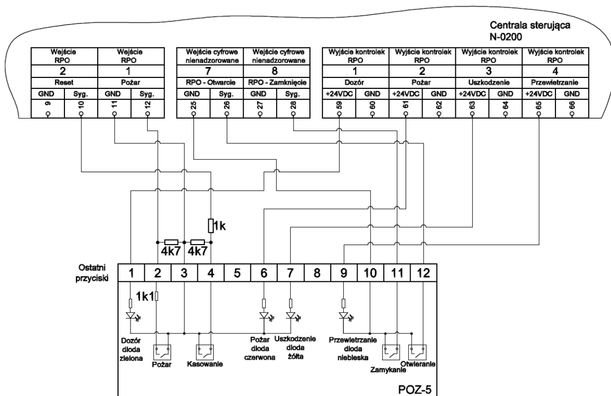
Rysunek 5.35. Schemat podłączenia przycisku POZ-4, POZ-5, POZ-6 dla jednej sztuki na linii.
