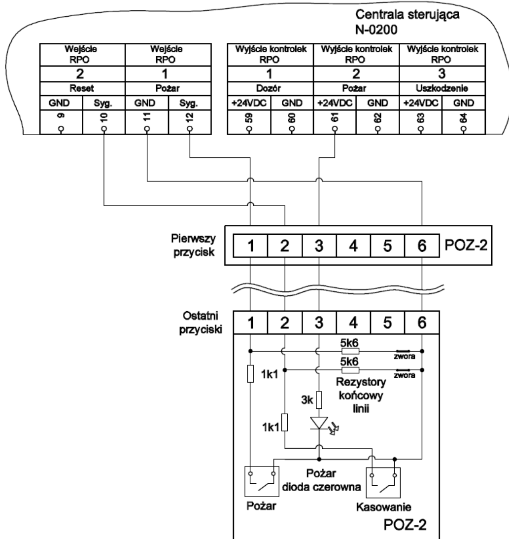
Rysunek 5.27. Schemat podłączenia przycisku POZ-2
