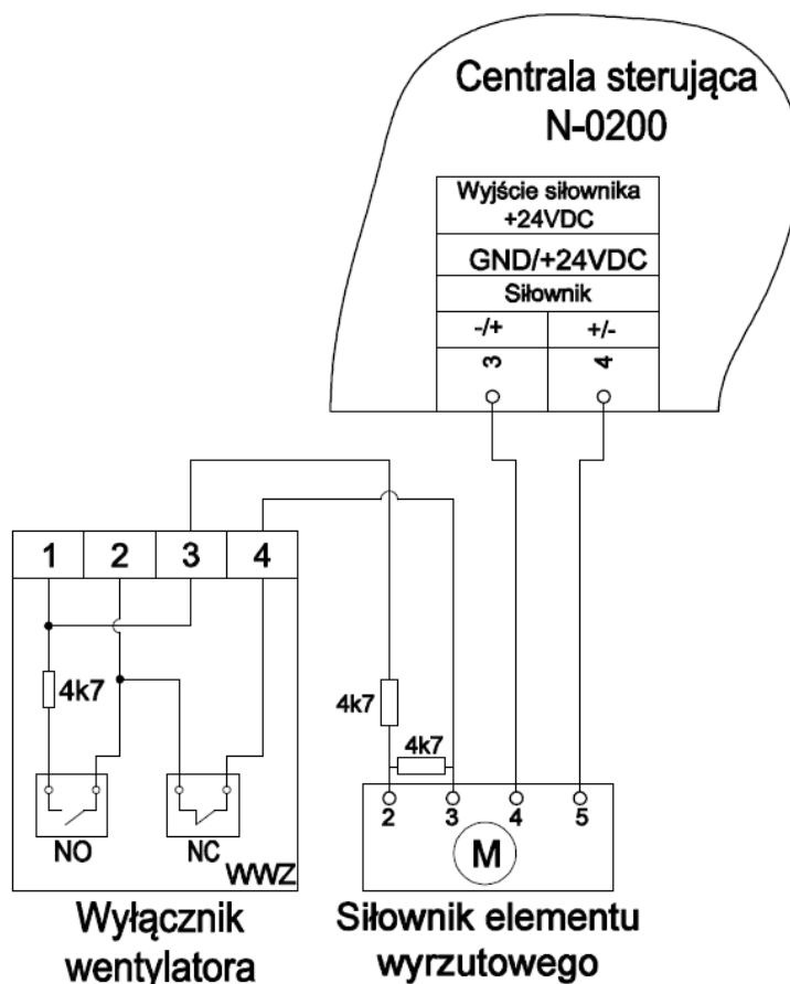
Rysunek 5.44. Schemat podłączenia zasilania siłownika kłapy
