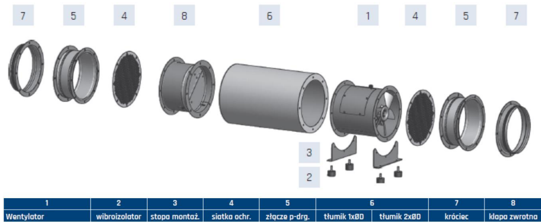
Rysunek 5.67. Schemat montażu kanałowych wentylatorów AFC
