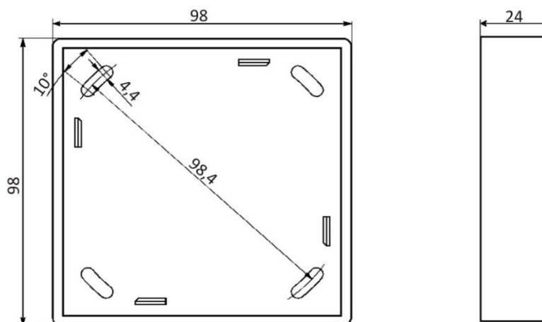
Rysunek 5.29. Wymiary i rozmieszczenie otworów montażowych ramki maskującej na przyciski POZ-1, POZ-2, POZ-3
