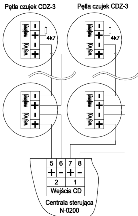
Rysunek 5.15. Schemat podłączenia czujek dymu CDZ-3
