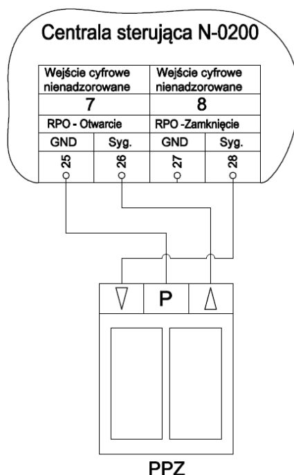
Rysunek 6.7. Schemat podłączenia przycisku przewietrzania
