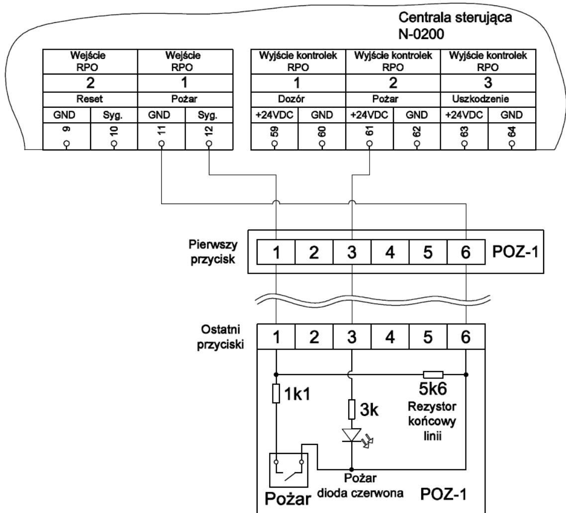
Rysunek 5.26. Schemat podłączenia przycisku POZ-1
