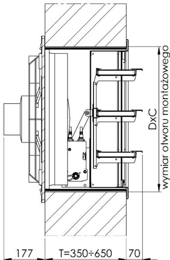
Rysunek 5.77. Zabudowa ZNZ
