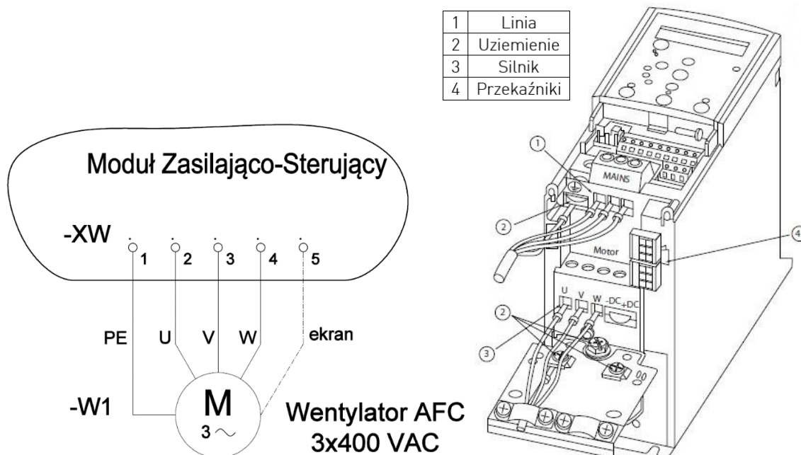
Rysunek 5.66. Schemat podłączenia wentylatora nawiewnego. Po lewej podłączenie przez zaciski śrubowe, po prawej bezpośrednio do przetwornicy częstotliwości.
