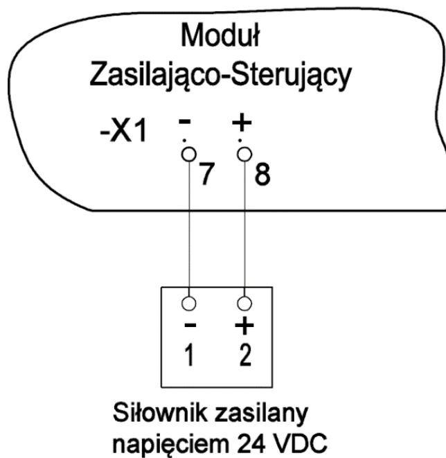
Rysunek 5.62. Schemat podłączenia siłownika czepni
