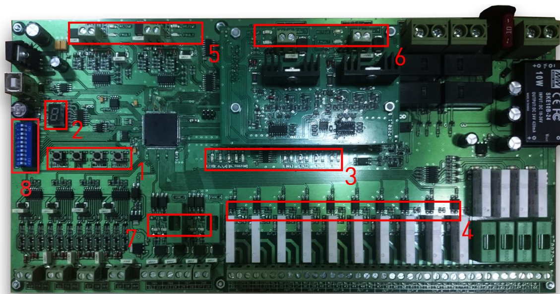
Rysunek 5.5. Opis płyty głównej N-0200
