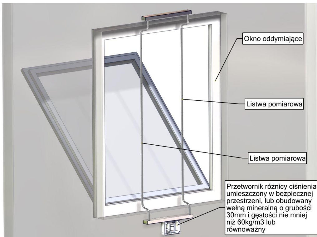
Rysunek 5.85. UPZ w otworze okna oddymiającego
