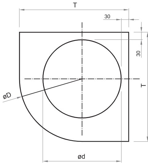
NAWIEWNIK NAROŻNY
