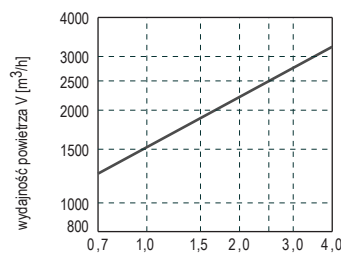
zasięg strugi L [m] dla v=0,25 m/s
