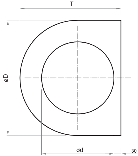
NAWIEWNIK PÓŁOKRĄGLY
