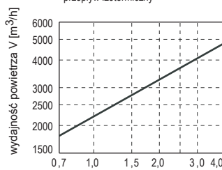
zasięg strugi L [m] dla v=0,25 m/s
