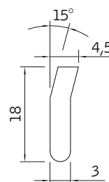
Nawiew kątowy KNK-T-al-15°
